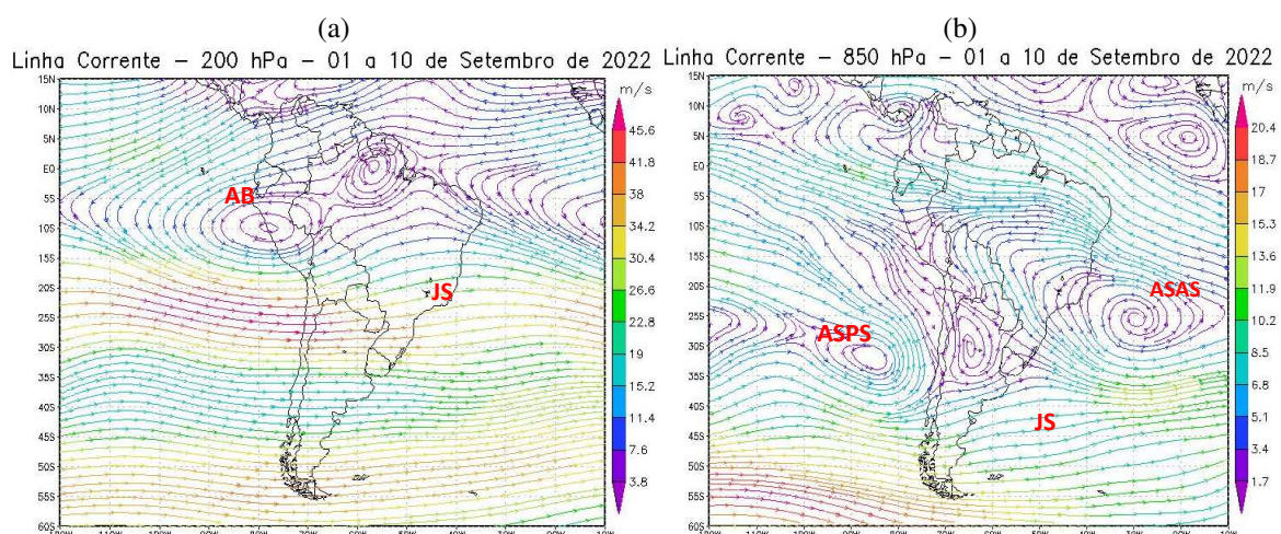
Figura 6 - Campos de Linha de Corrente 200 hPa. - (a) e 850 hPa. - (b), do 1º Decêndio de setembro de 2022; demonstrando interação entre os sistemas atmosféricos: Jato Subtropical (JS), Alta da Bolívia (AB), Anticiclone Subtropical do Atlântico Sul (ASAS) e o Anticiclone Subtropical do Pacífico Sul (ASPS).
