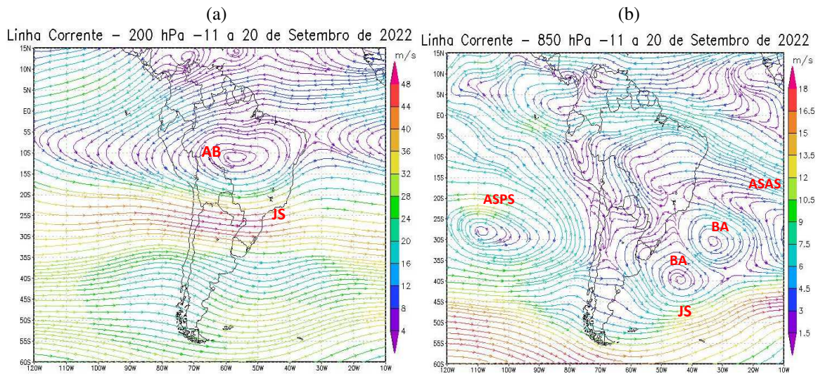
Figura 7 - Campos de Linha de Corrente 200 hPa. - (a) e 850 hPa. - (b), do 2º Decêndio de setembro de 2022; demonstrando interação entre os sistemas atmosféricos: Jato Subtropical (JS), Alta da Bolívia (AB), Anticiclone Subtropical do Atlântico Sul (ASAS) e o Anticiclone Subtropical do Pacífico Sul (ASPS) e Bloqueio Atmosférico (BA). FONTE - Dados: NOAA 2022.
