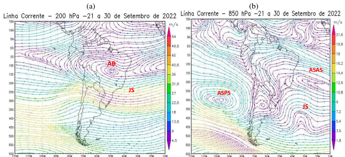
Figura 8 - Campos de Linha de Corrente 200 hPa. - (a) e 850 hPa. - (b), do 3º Decêndio de setembro de 2022; demonstrando interação entre os sistemas atmosféricos: Jato Subtropical (JS), Anticiclone Subtropical do Atlântico Sul (ASAS) e Anticiclone Subtropical do Pacífico Sul (ASPS),
