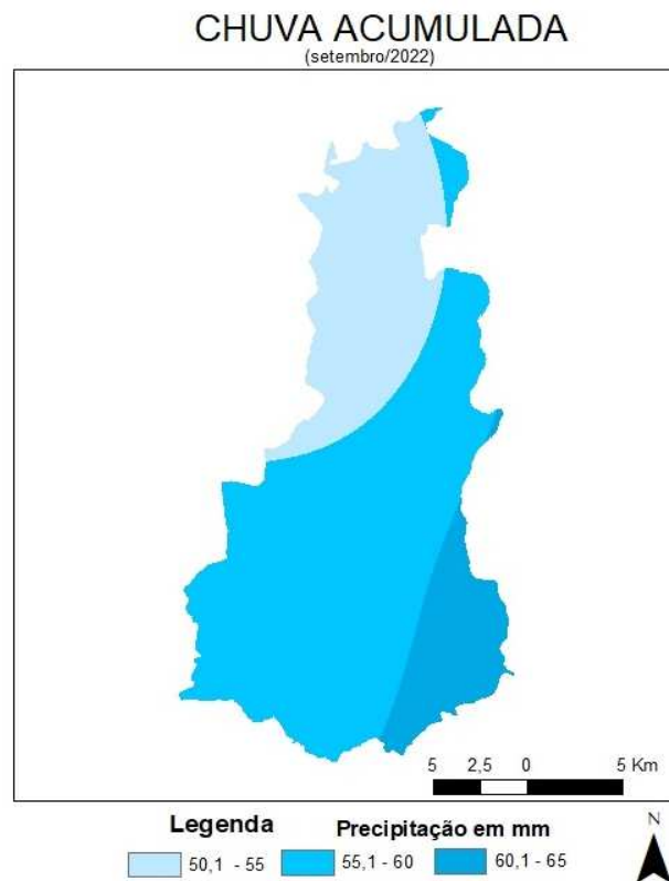
Figura 5 - Espacialização da Chuva da Acumulada em setembro de 2022. FONTE dos Dados: INMET e INPE
