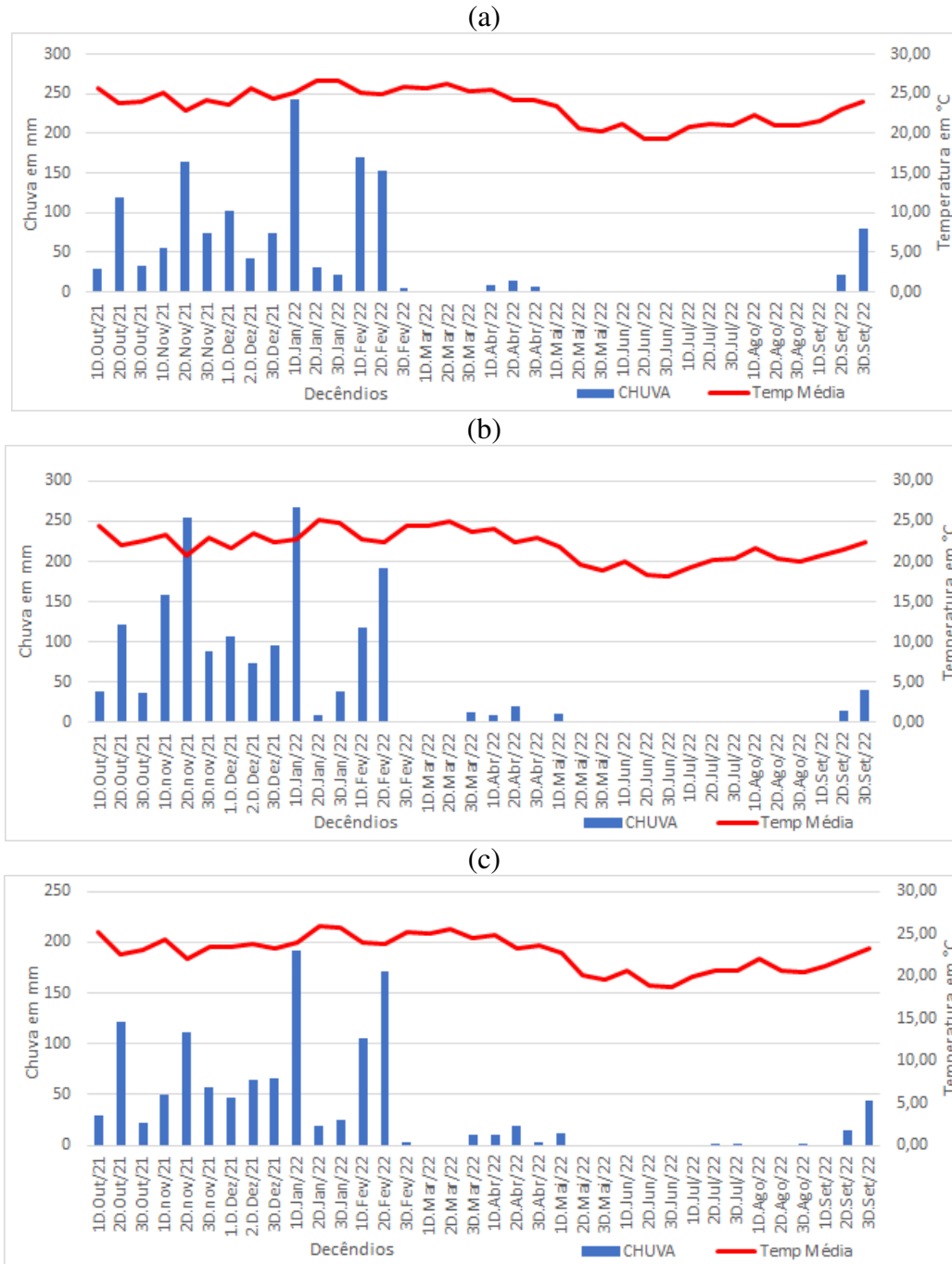
Figura 3: Histograma de Chuva e Temperatura: Caratinga (a); Timóteo (b) e PERD (c) – (outubro de 2021 a setembro de 2022).
