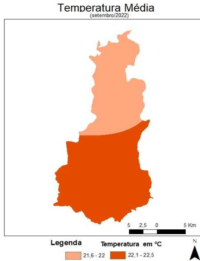
Figura 4 - Espacialização da Temperatura Média em setembro de 2022. FONTE dos Dados: INMET e INPE
