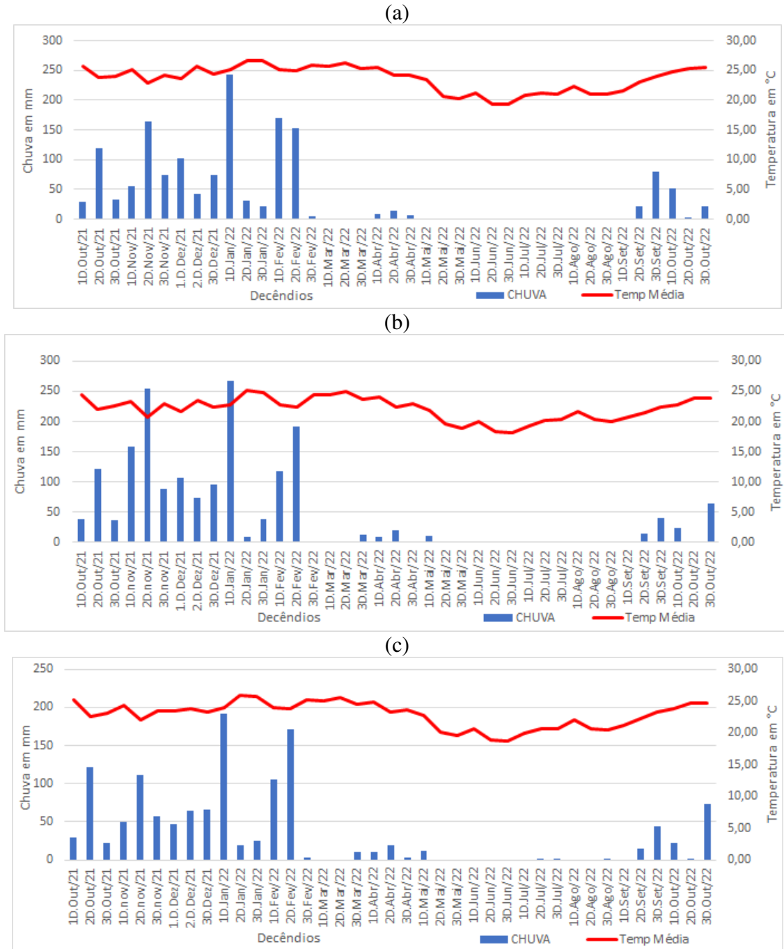
Figura 3: Histograma de Chuva e Temperatura: Caratinga (a); Timóteo (b) e PERD (c) – (outubro de 2021 a outubro de 2022).
