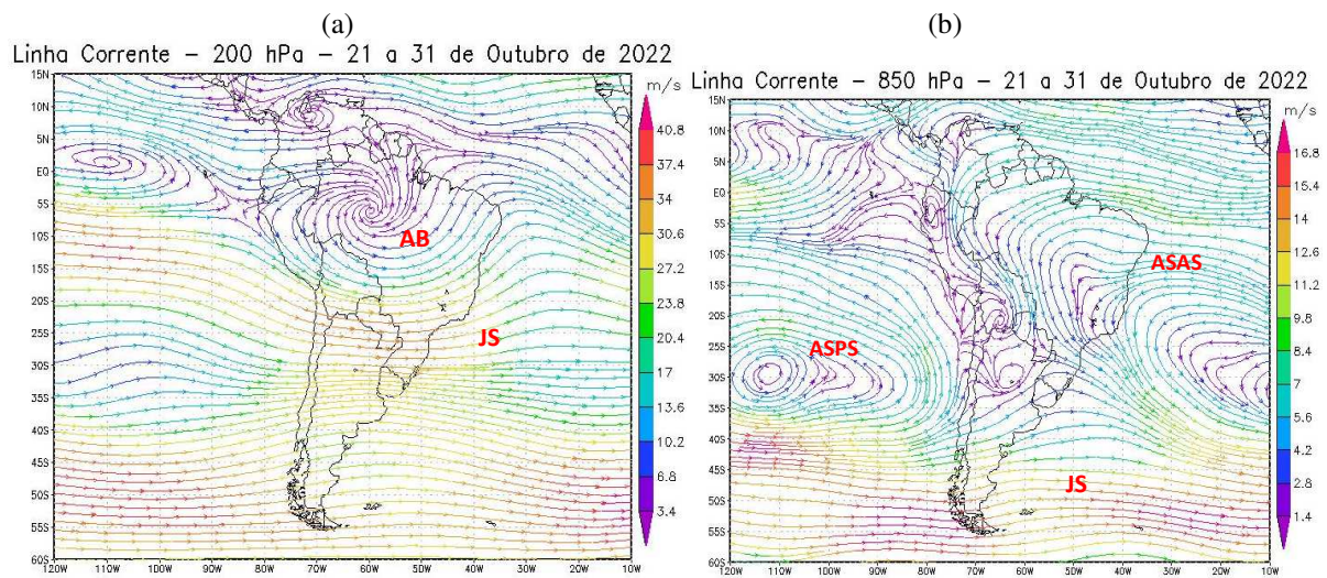
Figura 8 - Campos de Linha de Corrente 200 hPa. - (a) e 850 hPa. - (b), do 3º Decêndio de outubro de 2022; demonstrando interação entre os sistemas atmosféricos: Jato Subtropical (JS), Anticiclone Subtropical do Atlântico Sul (ASAS) e Anticiclone Subtropical do Pacífico Sul (ASPS),
