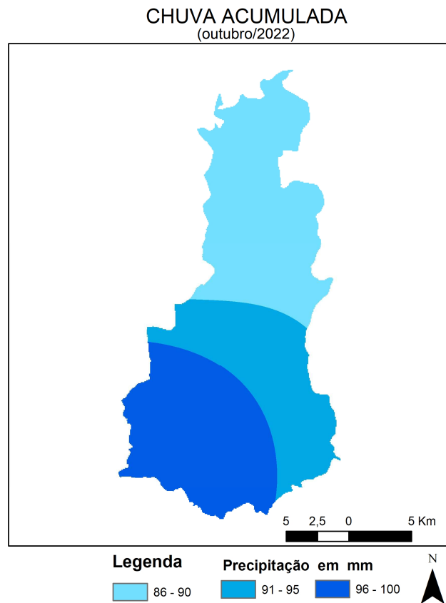
Figura 5 - Espacialização da Chuva da Acumulada em outubro de 2022. FONTE dos Dados: INMET e INPE
