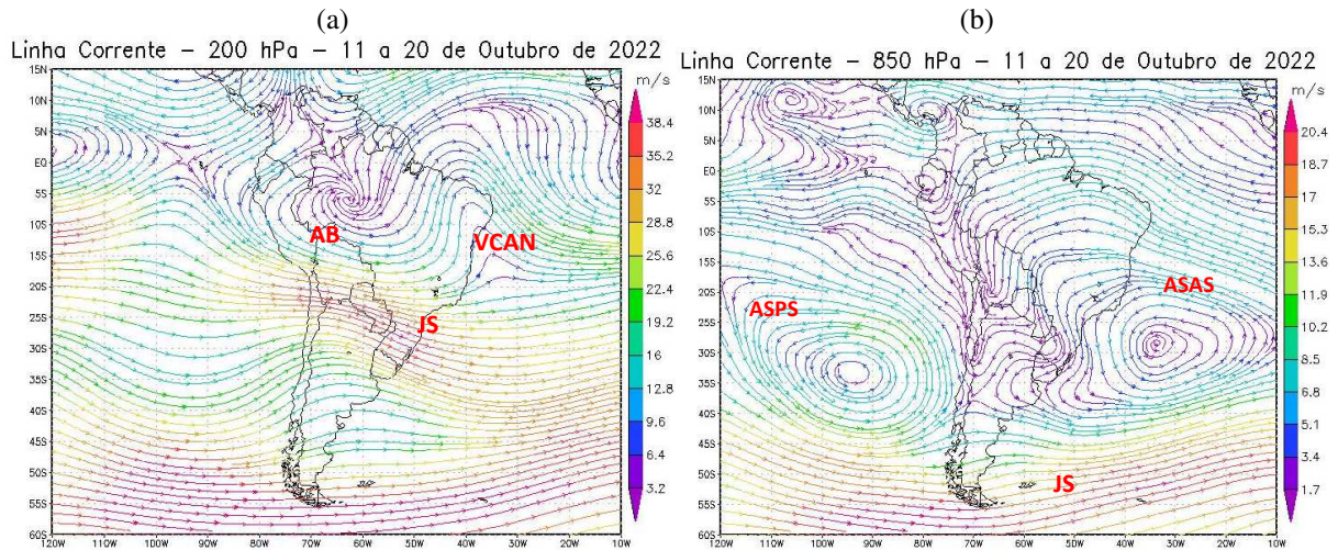
Figura 7 - Campos de Linha de Corrente 200 hPa. - (a) e 850 hPa. - (b), do 2º Decêndio de outubro de 2022; demonstrando interação entre os sistemas atmosféricos: Jato Subtropical (JS), Alta da Bolívia (AB), Vórtice Ciclônico de Altos Níveis (VCAN), Anticiclone Subtropical do Atlântico Sul (ASAS) e o Anticiclone Subtropical do Pacífico Sul (ASPS) e Bloqueio Atmosférico (BA).
