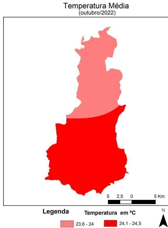
Figura 4 - Espacialização da Temperatura Média em outubro de 2022. FONTE dos Dados: INMET e INPE
