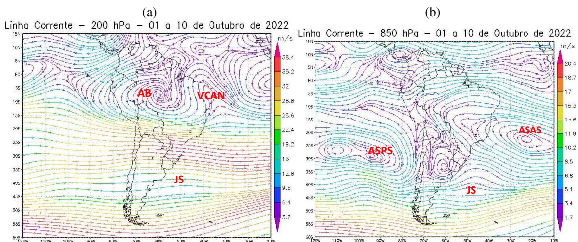
Figura 6 - Campos de Linha de Corrente 200 hPa. - (a) e 850 hPa. - (b), do 1º Decêndio de outubro de 2022; demonstrando interação entre os sistemas atmosféricos: Jato Subtropical (JS), Alta da Bolívia (AB), Vórtice Ciclônico de Altos Níveis (VCAN), Anticiclone Subtropical do Atlântico Sul (ASAS) e o Anticiclone Subtropical do Pacífico Sul (ASPS).
