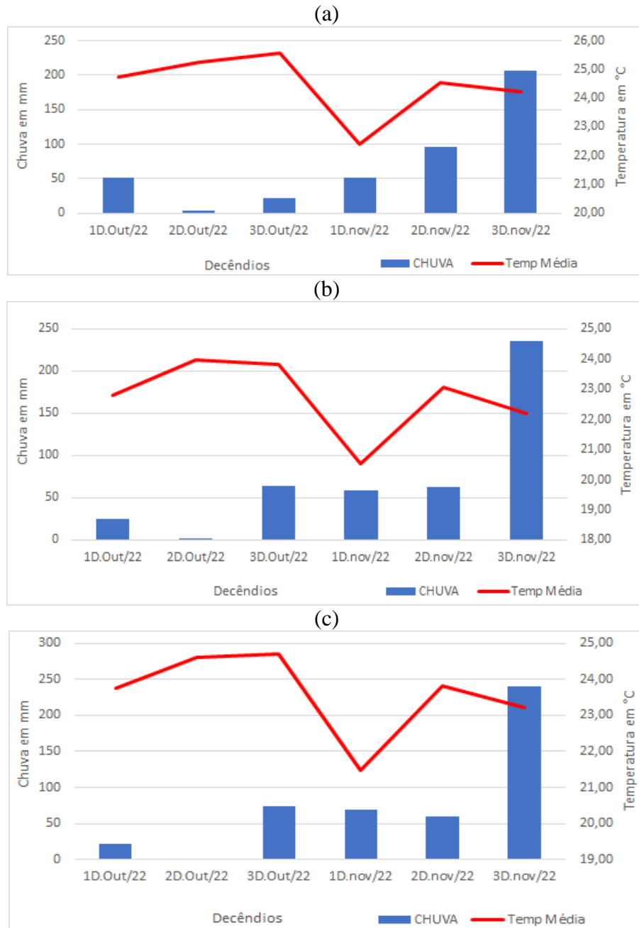
Figura 3: Histograma de Chuva e Temperatura: Caratinga (a); Timóteo (b) e PERD (c) – (outubro a novembro de 2022).
