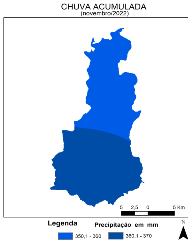
Figura 5 - Espacialização da Chuva da Acumulada em novembro de 2022. FONTE dos Dados: INMET e INPE
