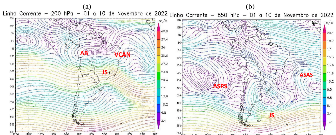
Figura 6 - Campos de Linha de Corrente 200 hPa. - (a) e 850 hPa. - (b), do 1º Decêndio de novembro de 2022; demonstrando interação entre os sistemas atmosféricos: Jato Subtropical (JS), Alta da Bolívia (AB), Vórtice Ciclônico de Altos Níveis (VCAN), Anticiclone Subtropical do Atlântico Sul (ASAS) e o Anticiclone Subtropical do Pacífico Sul (ASPS).
