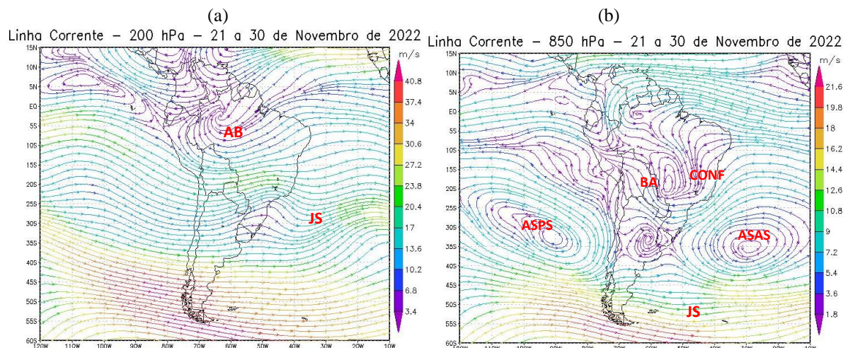
Figura 8 - Campos de Linha de Corrente 200 hPa. - (a) e 850 hPa. - (b), do 3º Decêndio de novembro de 2022; demonstrando interação entre os sistemas atmosféricos: Jato Subtropical (JS), Alta da Bolívia (AB), Anticiclone Subtropical do Atlântico Sul (ASAS), Anticiclone Subtropical do Pacífico Sul (ASPS) e Bloqueio Atmosférico (BA).
