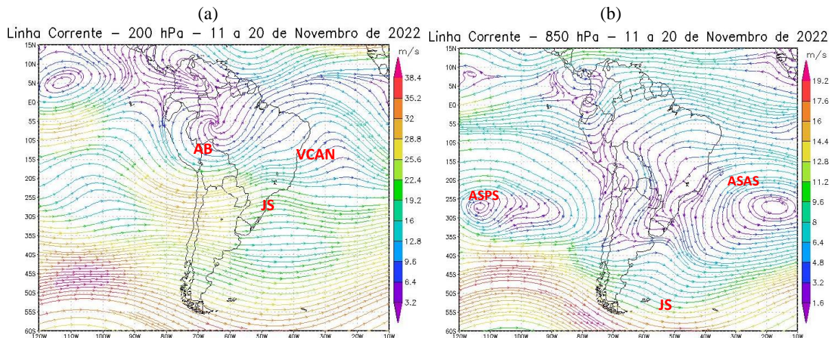
Figura 7 - Campos de Linha de Corrente 200 hPa. - (a) e 850 hPa. - (b), do 2º Decêndio de novembro de 2022; demonstrando interação entre os sistemas atmosféricos: Jato Subtropical (JS), Alta da Bolívia (AB), Vórtice Ciclônico de Altos Níveis (VCAN), Anticiclone Subtropical do Atlântico Sul (ASAS) e o Anticiclone Subtropical do Pacífico Sul (ASPS) e Bloqueio Atmosférico (BA).
