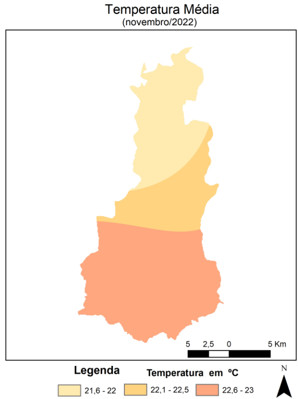
Figura 4 - Espacialização da Temperatura Média em novembro de 2022. FONTE dos Dados: INMET e INPE
