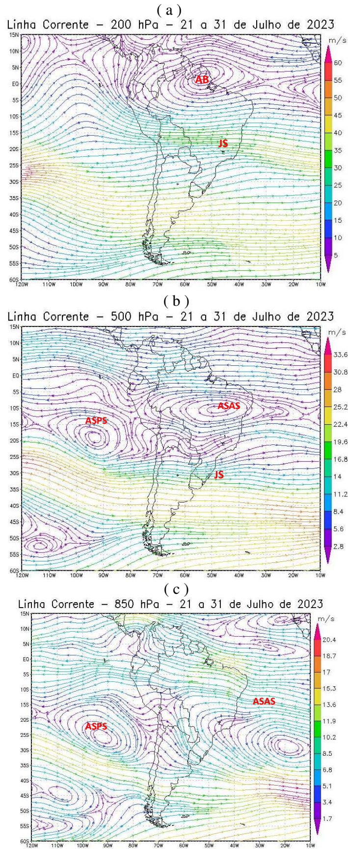
Figura 8 - Campos de Linha de Corrente 200 hPa- (a), 500 hPa - (b) e 850 hPa – (c), do 3º Decêndio de julho de 2023; demonstrando interação entre os sistemas atmosféricos: Jato Subtropical (JS), Alta da Bolívia (AB), Anticiclone Subtropical do Atlântico Sul (ASAS) e Anticiclone Subtropical do Pacífico Sul (ASPS). FONTE - Dados: NOAA 2023.
