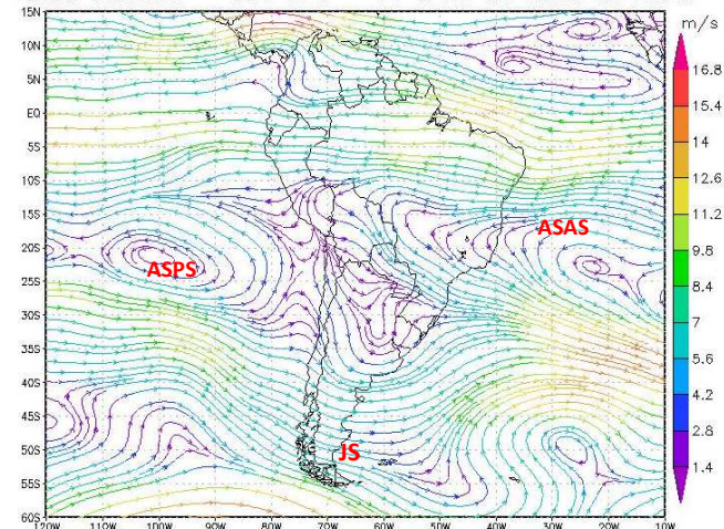
Figura 7 - Campos de Linha de Corrente 200 hPa. - (a), 500 hPa. - (b) e 850 hPa - (c), do 2º Decêndio de julho de 2023; demonstrando interação entre os sistemas atmosféricos: Jato Subtropical (JS), Alta da Bolívia (AB), Bloqueio Atmosférico (BA), Anticiclone Subtropical do Atlântico Sul (ASAS) e o Anticiclone Subtropical do Pacífico Sul (ASPS). FONTE - Dados: NOAA 2023.
