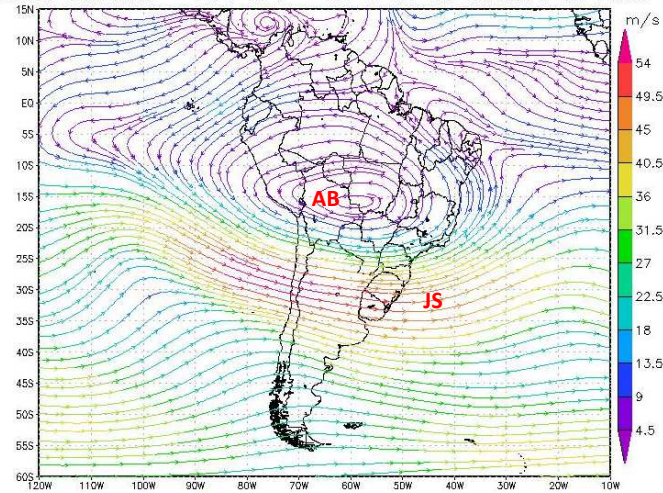
(b) Linha Corrente – 500 hPa – 21 a 31 de Outubro de 2023
