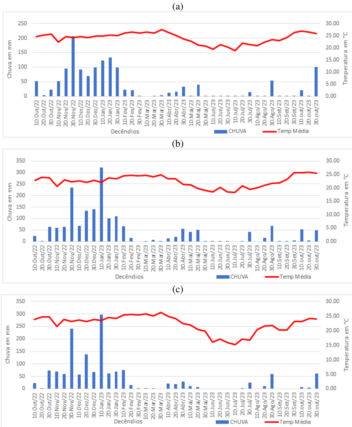
Figura 3: Histograma de Chuva e Temperatura: Caratinga (a); Timóteo (b) e PERD (c) – (outubro de 2022 a outubro de 2023).
