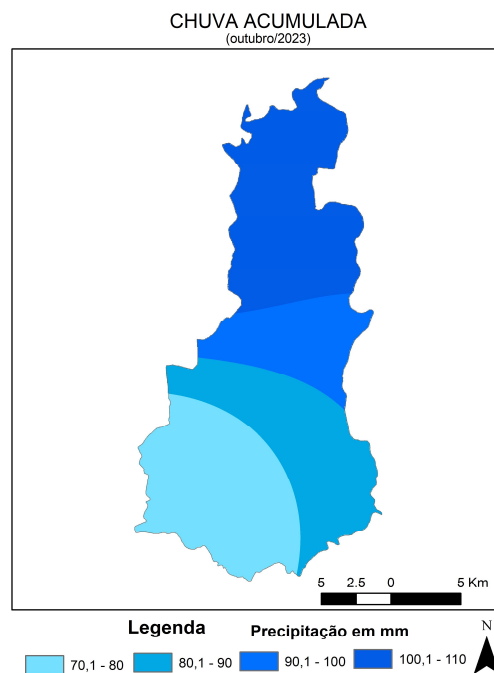
Figura 5 - Espacialização da Chuva da Acumulada em outubro de 2023. FONTE dos Dados: INMET e INPE
