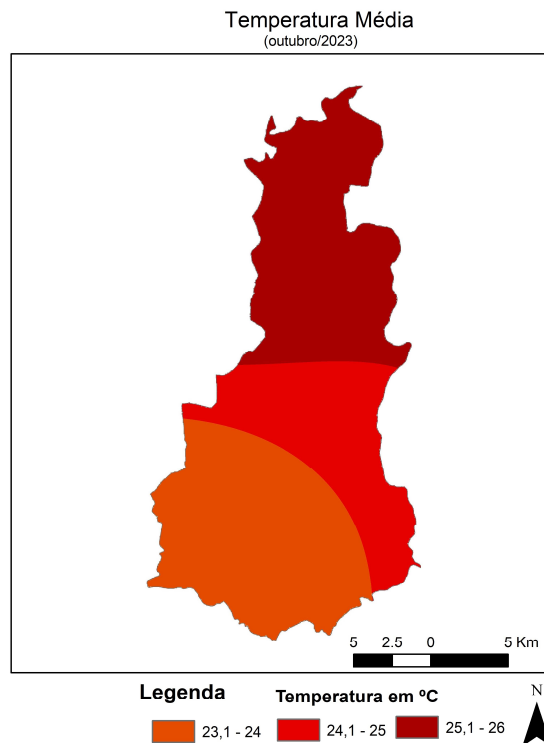
Figura 4 - Espacialização da Temperatura Média em outubro de 2023. FONTE dos Dados: INMET e INPE
