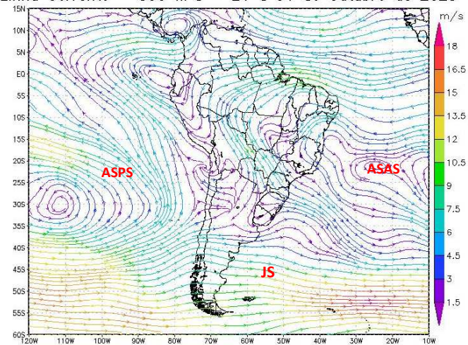
(c) Linha Corrente – 850 hPa – 21 a 31 de Outubro de 2023
