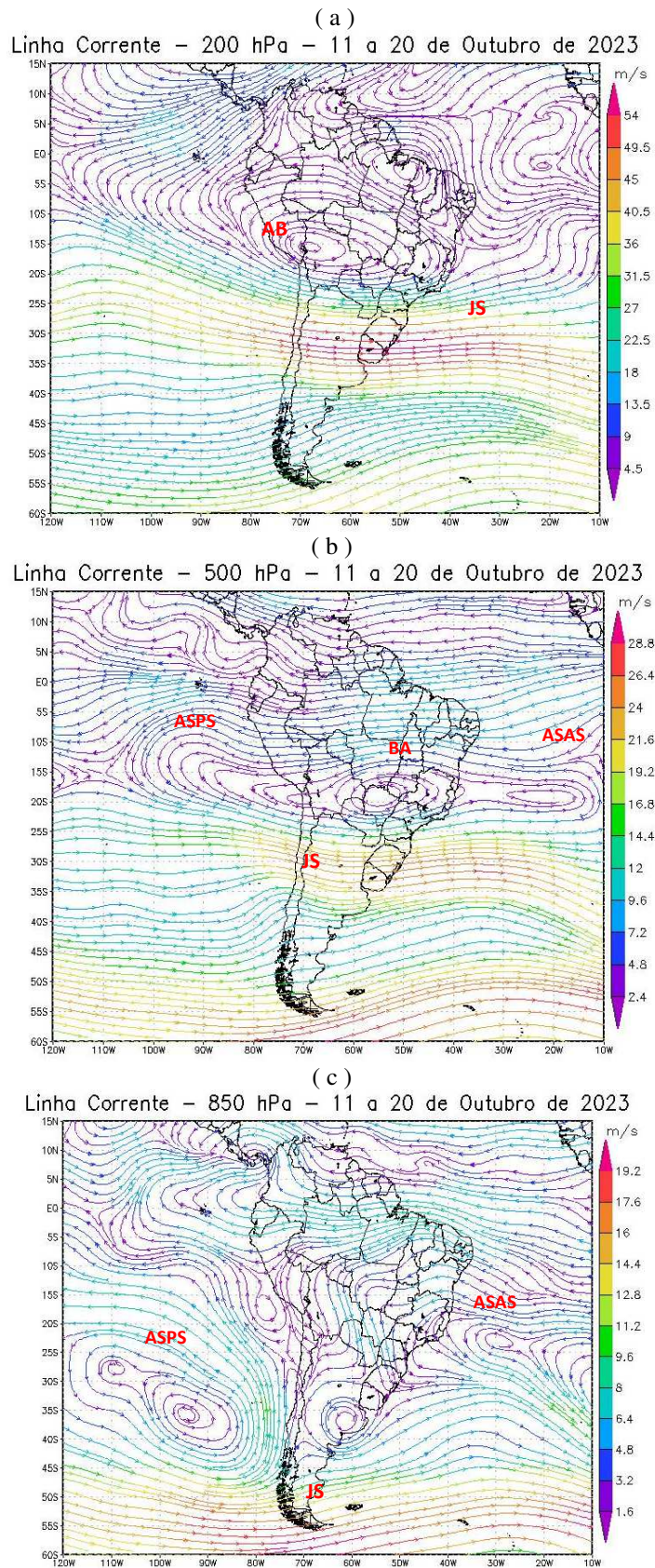
Figura 7 - Campos de Linha de Corrente 200 hPa. - (a), 500 hPa. - (b) e 850 hPa - (c), do 2º Decêndio de outubro de 2023; demonstrando interação entre os sistemas atmosféricos: Jato Subtropical (JS), Alta da Bolívia (AB), Bloqueio Atmosférico (BA), Anticiclone Subtropical do Atlântico Sul (ASAS) e o Anticiclone Subtropical do Pacífico Sul (ASPS). FONTE - Dados: NOAA 2023.
