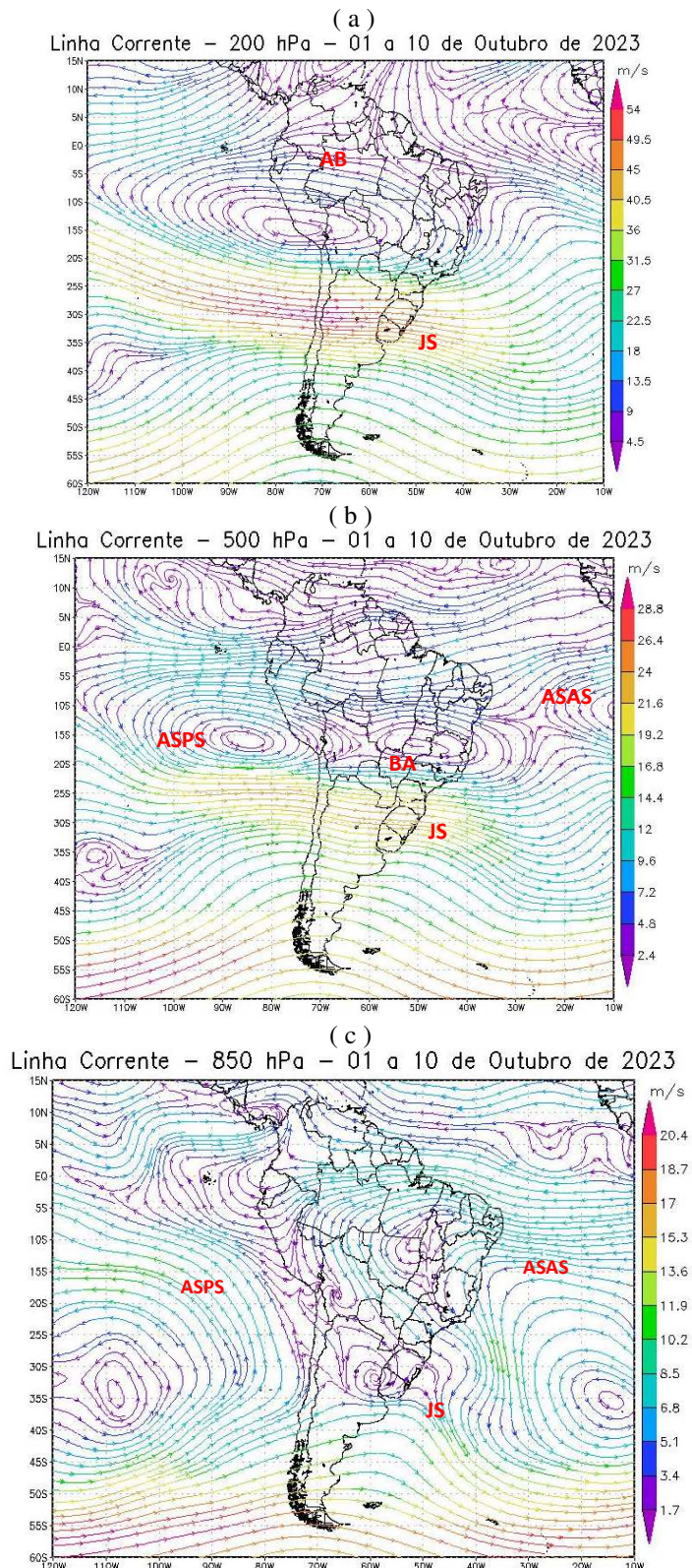
Figura 6 - Campos de Linha de Corrente 200 hPa. - (a), 500 hPa. - (b) e 850 hPa - (c), do 1º Decêndio de outubro de 2023; demonstrando interação entre os sistemas atmosféricos: Jato Subtropical (JS), Alta da Bolívia (AB), Bloqueio Atmosférico (BA), Anticiclone Subtropical do Atlântico Sul (ASAS) e o Anticiclone Subtropical do Pacífico Sul (ASPS). FONTE - Dados: NOAA 2023.
