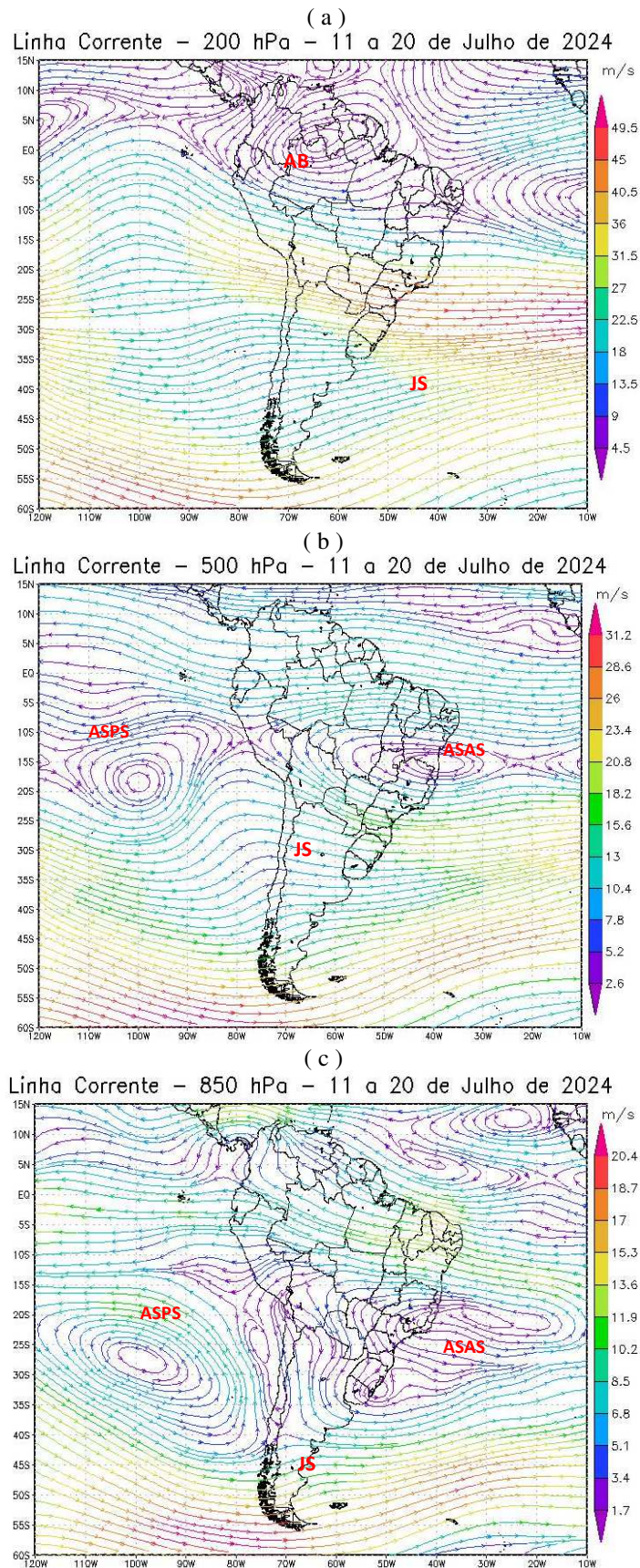
Figura 7 - Campos de Linha de Corrente 200 hPa. - (a), 500 hPa. - (b) e 850 hPa - (c), do 2º Decêndio de julho de 2024; demonstrando interação entre os sistemas atmosféricos: Jato Subtropical (JS), Alta da Bolívia (AB), Anticiclone Subtropical do Atlântico Sul (ASAS) e o Anticiclone Subtropical do Pacífico Sul (ASPS). FONTE - Dados: NOAA 2024.
