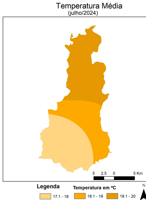
Figura 4 - Espacialização da Temperatura Média em julho de 2024. FONTE dos Dados: INMET e INPE CLIMAPERD – v. 04, n. 08 – Jul/2024
