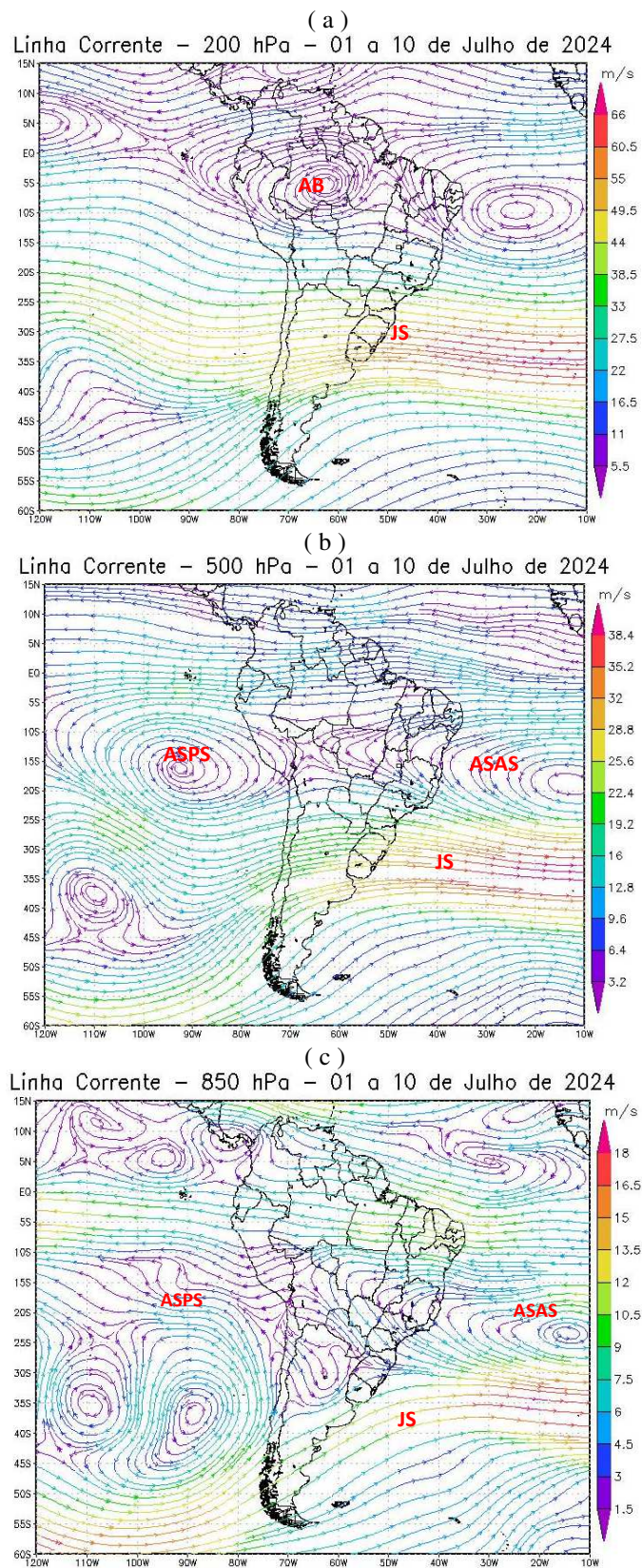
Figura 6 - Campos de Linha de Corrente 200 hPa. - (a), 500 hPa - (b) e 850 hPa - (c), do 1º Decêndio de julho de 2024; demonstrando interação entre os sistemas atmosféricos: Jato Subtropical (JS), Alta da Bolívia (AB), Anticiclone Subtropical do Atlântico Sul (ASAS) e o Anticiclone Subtropical do Pacífico Sul (ASPS). FONTE - Dados: NOAA 2024.
