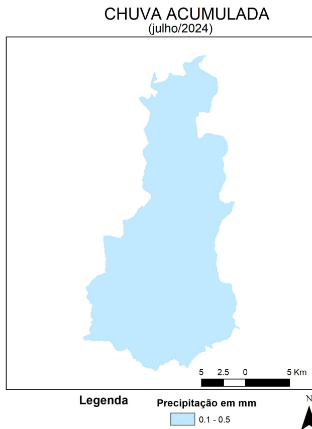
Figura 5 - Espacialização da Chuva da Acumulada em julho de 2024. FONTE dos Dados: INMET e INPE
