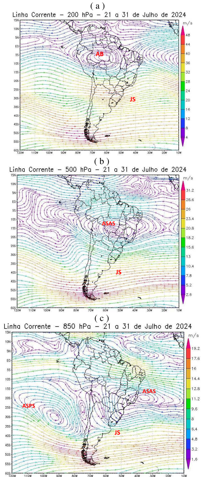
Figura 8 - Campos de Linha de Corrente 200 hPa- (a), 500 hPa - (b) e 850 hPa – (c), do 3º Decêndio de julho de 2024; demonstrando interação entre os sistemas atmosféricos: Jato Subtropical (JS), Alta da Bolívia (AB), Anticiclone Subtropical do Atlântico Sul (ASAS) e Anticiclone Subtropical do Pacífico Sul (ASPS).
