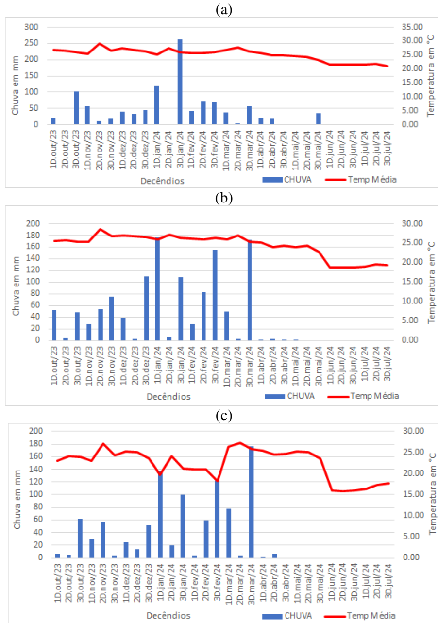
Figura 3: Histograma de Chuva e Temperatura: Caratinga (a); Timóteo (b) e PERD (c) – (outubro de 2023 a julho de 2024).
