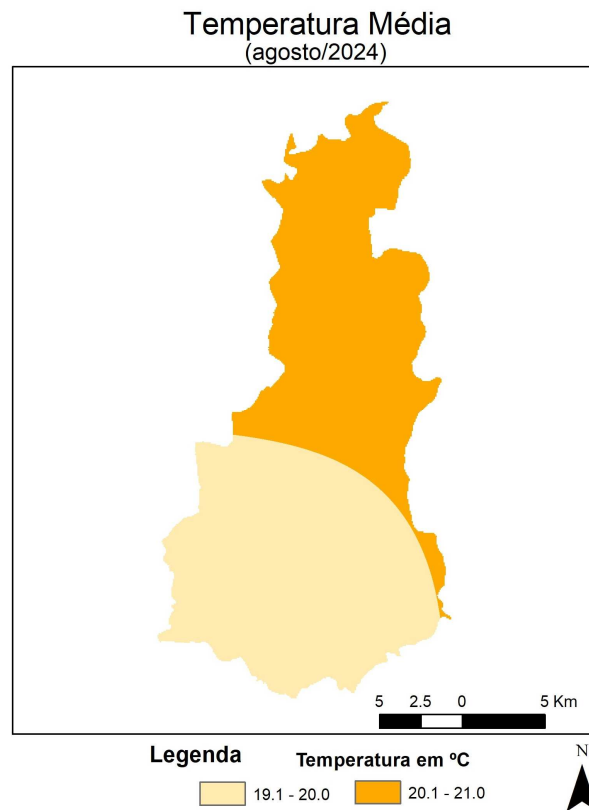
Figura 4 - Espacialização da Temperatura Média em agosto de 2024. FONTE dos Dados: INMET e INPE
