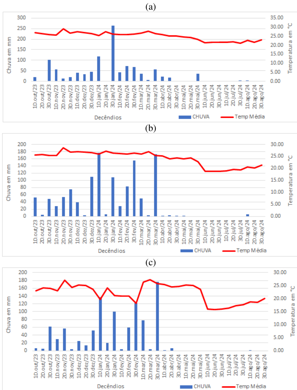
Figura 3: Histograma de Chuva e Temperatura: Caratinga (a); Timóteo (b) e PERD (c) – (outubro de 2023 a agosto de 2024).
