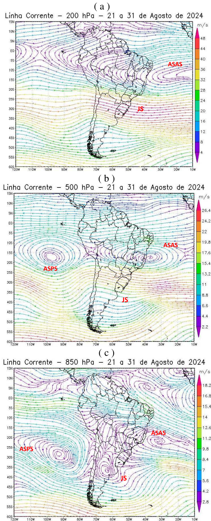
Figura 8 - Campos de Linha de Corrente 200 hPa- (a), 500 hPa - (b) e 850 hPa – (c), do 3º Decêndio de agosto de 2024; demonstrando interação entre os sistemas atmosféricos: Jato Subtropical (JS), Anticiclone Subtropical do Atlântico Sul (ASAS) e Anticiclone Subtropical do Pacífico Sul (ASPS).
