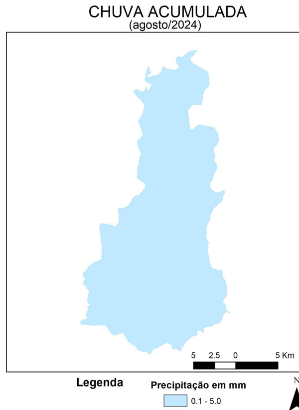
Figura 5 - Espacialização da Chuva da Acumulada em agosto de 2024. FONTE dos Dados: INMET e INPE
