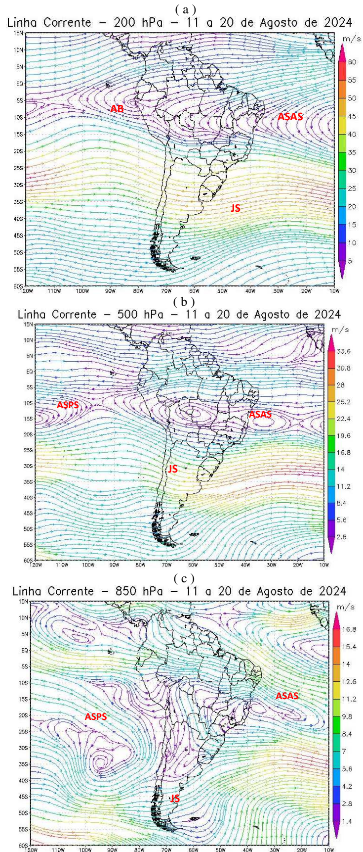
Figura 7 - Campos de Linha de Corrente 200 hPa. - (a), 500 hPa. - (b) e 850 hPa – (c), do 2º Decêndio de agosto de 2024; demonstrando interação entre os sistemas atmosféricos: Jato Subtropical (JS), Alta da Bolívia (AB), Anticiclone Subtropical do Atlântico Sul (ASAS) e o Anticiclone Subtropical do Pacífico Sul (ASPS). FONTE - Dados: NOAA 2024.
