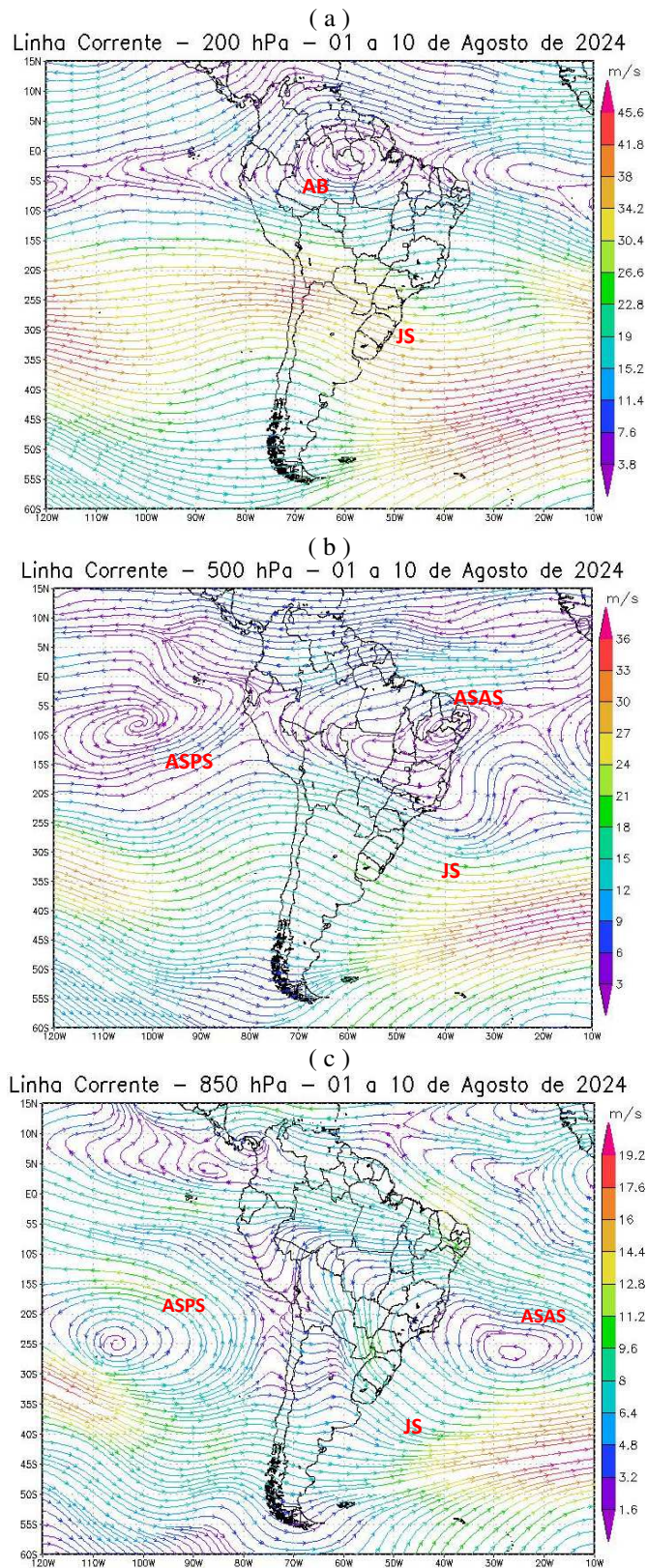
Figura 6 - Campos de Linha de Corrente 200 hPa. - (a), 500 hPa. - (b) e 850 hPa – (c), do 1º Decêndio de agosto de 2024; demonstrando interação entre os sistemas atmosféricos: Jato Subtropical (JS), Alta da Bolívia (AB), Anticiclone Subtropical do Atlântico Sul (ASAS) e o Anticiclone Subtropical do Pacífico Sul (ASPS). FONTE - Dados: NOAA 2024.
