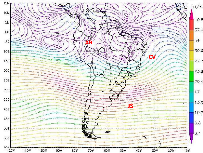
(b) Linha Corrente – 500 hPa – 11 a 20 de Outubro de 2024
