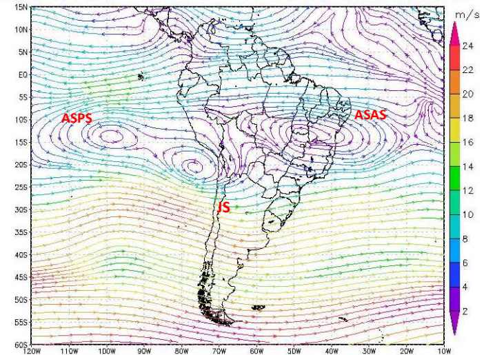
(c) Linha Corrente – 850 hPa – 11 a 20 de Outubro de 2024
