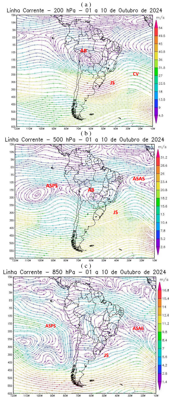
Figura 6 - Campos de Linha de Corrente 200 hPa. - (a), 500 hPa. - (b) e 850 hPa - (c), do 1º Decêndio de outubro de 2024; demonstrando interação entre os sistemas atmosféricos: Jato Subtropical (JS), Alta da Bolívia (AB), Cavado (CV), Anticiclone Subtropical do Atlântico Sul (ASAS) e o Anticiclone Subtropical do Pacífico Sul (ASPS). FONTE - Dados: NOAA 2024.
