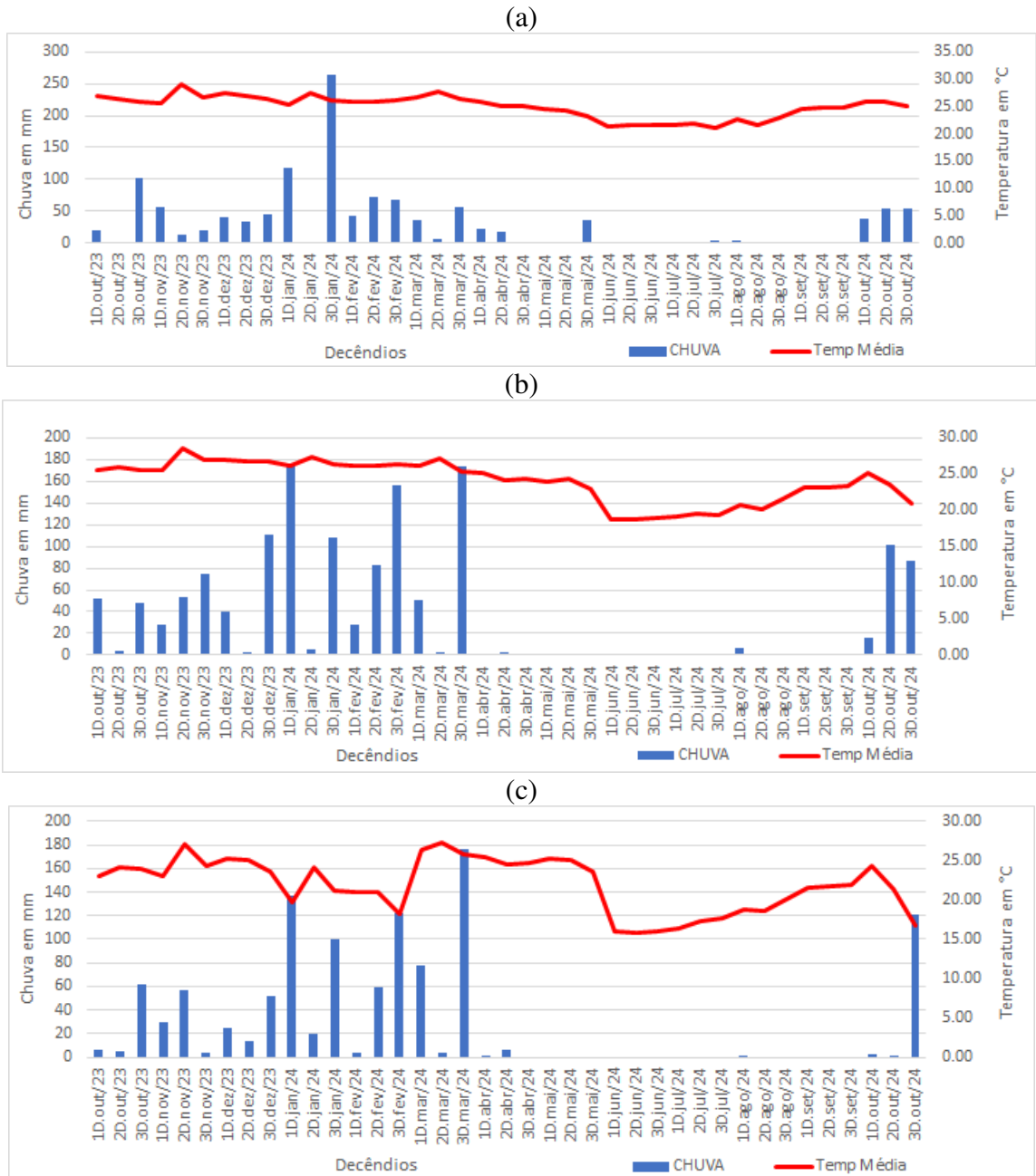
Figura 3: Histograma de Chuva e Temperatura: Caratinga (a); Timóteo (b) e PERD (c) – (outubro de 2023 a outubro de 2024).
