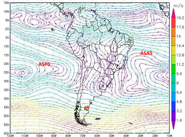
Figura 7 - Campos de Linha de Corrente 200 hPa. - (a), 500 hPa. - (b) e 850 hPa - (c), do 2º Decêndio de outubro de 2024; demonstrando interação entre os sistemas atmosféricos: Jato Subtropical (JS), Alta da Bolívia (AB), Cavado (CV), Anticiclone Subtropical do Atlântico Sul (ASAS) e o Anticiclone Subtropical do Pacífico Sul (ASPS). FONTE - Dados: NOAA 2024.
