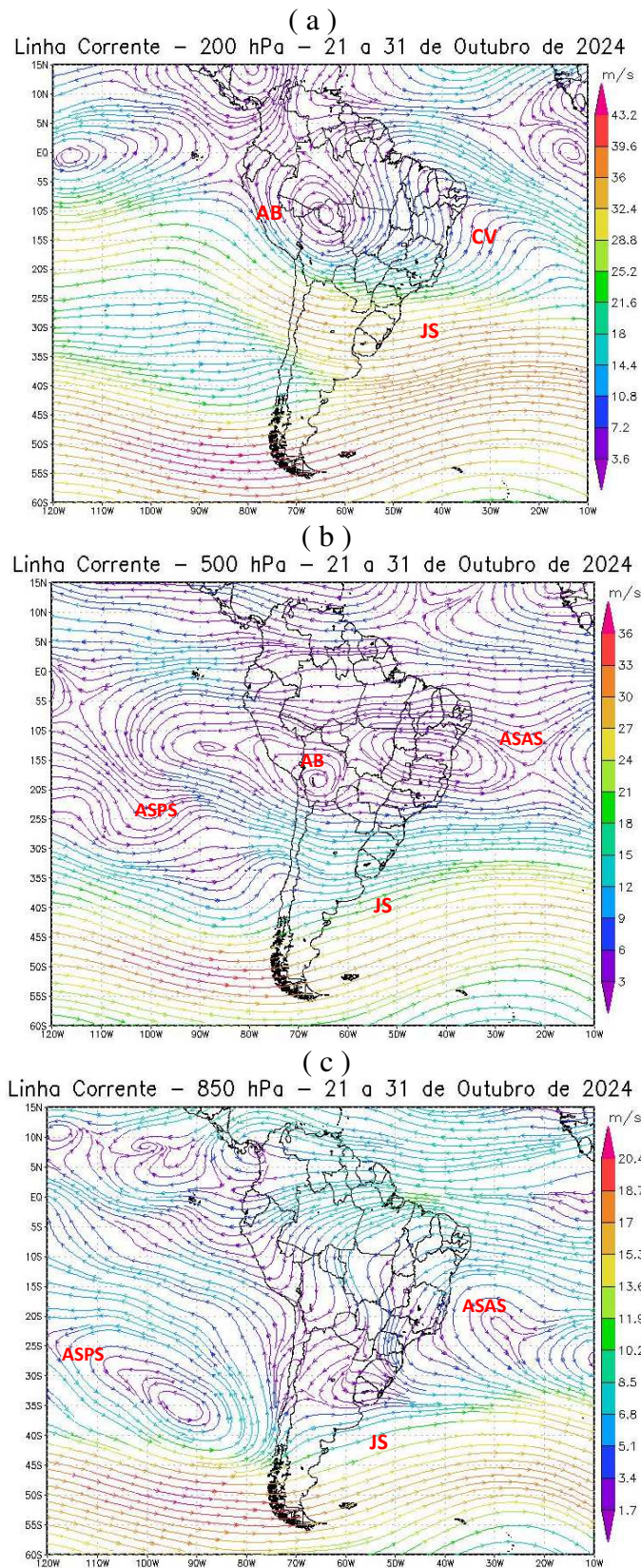
Figura 8 - Campos de Linha de Corrente 200 hPa- (a), 500 hPa- (b) e 850 hPa – (c), do 3º Decêndio de outubro de 2024; demonstrando interação entre os sistemas atmosféricos: Jato Subtropical (JS), Alta da Bolívia (AB), Cavado (CV), Anticiclone Subtropical do Atlântico Sul (ASAS) e Anticiclone Subtropical do Pacífico Sul (ASPS).
