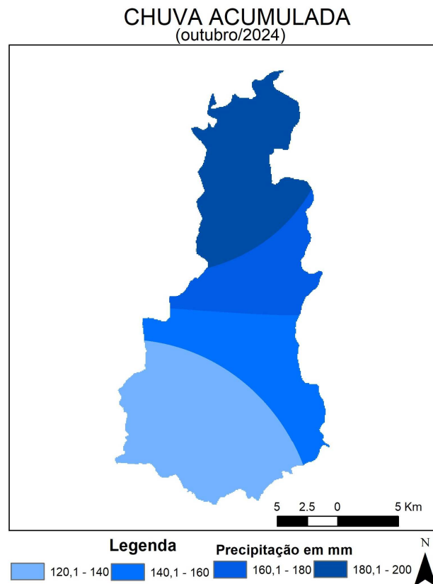
Figura 5 - Espacialização da Chuva da Acumulada em outubro de 2024. FONTE dos Dados: INMET e INPE
