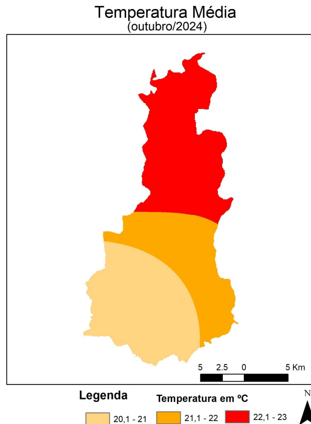
Figura 4 - Espacialização da Temperatura Média em outubro de 2024. FONTE dos Dados: INMET e INPE
