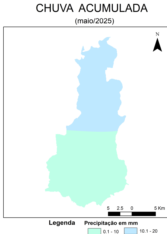
Figura 5 - Espacialização da Chuva da Acumulada em maio de 2025. FONTE dos Dados: INMET e INPE
