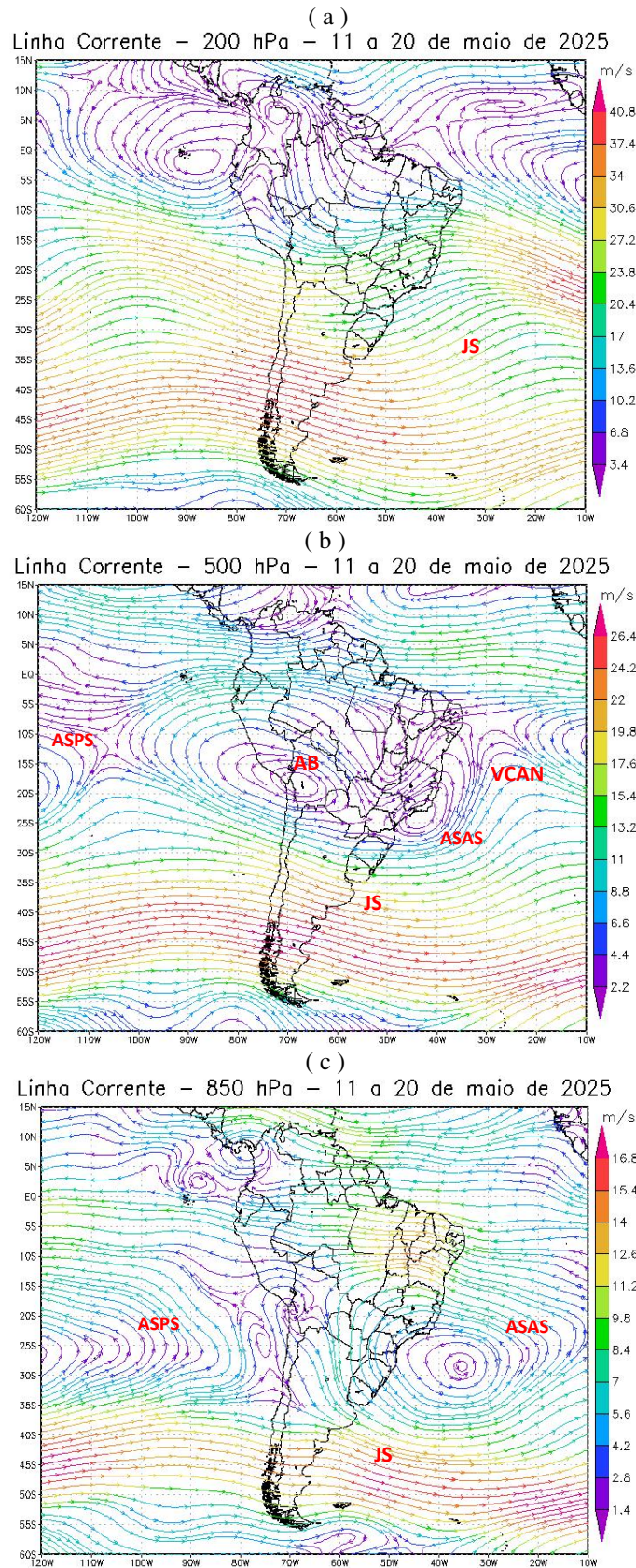
Figura 7 - Campos de Linha de Corrente 200 hPa. - (a), 500 hPa. - (b) e 850 hPa – (c), do 2º Decêndio de maio de 2025; demonstrando interação entre os sistemas atmosféricos: Jato Subtropical (JS), Alta da Bolívia (AB), Vórtice Ciclônico de Altos Níveis (VCAN), Anticiclone Subtropical do Atlântico Sul (ASAS) e o Anticiclone Subtropical do Pacífico Sul (ASPS).
