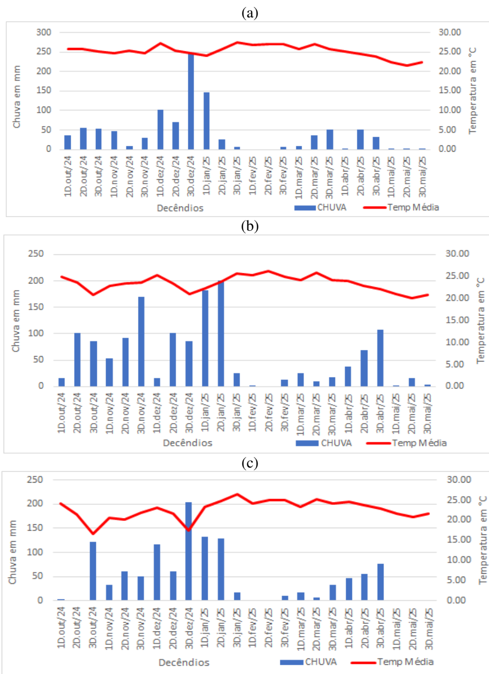
Figura 3: Histograma de Chuva e Temperatura: Caratinga (a); Timóteo (b) e PERD (c) – (outubro de 2024 a maio de 2025).
