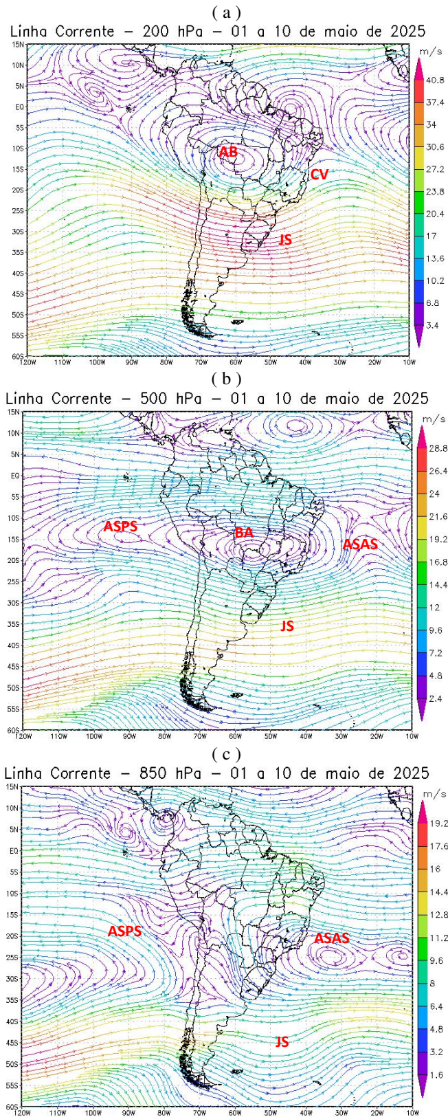
Figura 6 - Campos de Linha de Corrente 200 hPa. - (a), 500 hPa. - (b) e 850 hPa – (c), do 1º Decêndio de maio de 2025; demonstrando interação entre os sistemas atmosféricos: Jato Subtropical (JS), Alta da Bolívia (AB), Cavado (CV), Bloqueio Atmosférico (BA), Anticiclone Subtropical do Atlântico Sul (ASAS) e o Anticiclone Subtropical do Pacífico Sul (ASPS).
