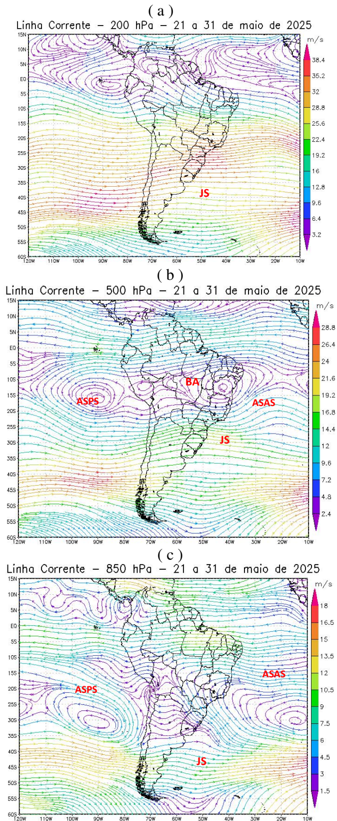
Figura 8 - Campos de Linha de Corrente 200 hPa - (a), 500 hPa - (b) e 850 hPa - (c), do 3º Decêndio de maio de 2025; demonstrando interação entre os sistemas atmosféricos: Jato Subtropical (JS), Bloqueio Atmosférico (BA) Anticiclone Subtropical do Atlântico Sul (ASAS) e Anticiclone Subtropical do Pacífico Sul (ASPS). FONTE - Dados: NOAA 2025.
