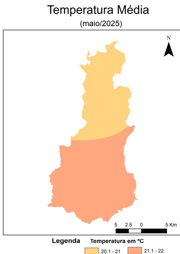
Figura 4 - Espacialização da Temperatura Média em maio de 2025. FONTE dos Dados: INMET e INPE
