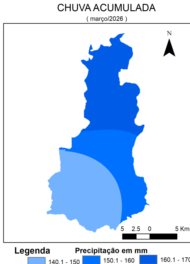
Figura 5 - Espacialização da Chuva da Acumulada em março de 2026. FONTE dos Dados: INMET e CEMADEN
