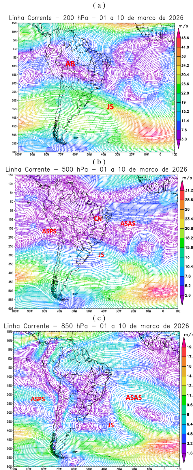
Figura 6 - Campos de Linha de Corrente 200 hPa (a), 500 hPa (b) e 850 hPa (c), do 1º Decêndio de março de 2026; demonstrando interação entre os sistemas atmosféricos: Jato Subtropical (JS), Alta da Bolívia (AB), Cavado do Nordeste (CN), Anticiclone Subtropical do Atlântico Sul (ASAS) e o Anticiclone Subtropical do Pacífico Sul (ASPS).
