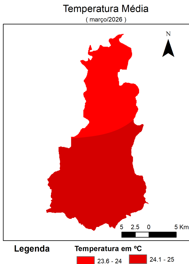
Figura 4 - Espacialização da Temperatura Média em março de 2026. FONTE dos Dados: INMET e CEMADEN
