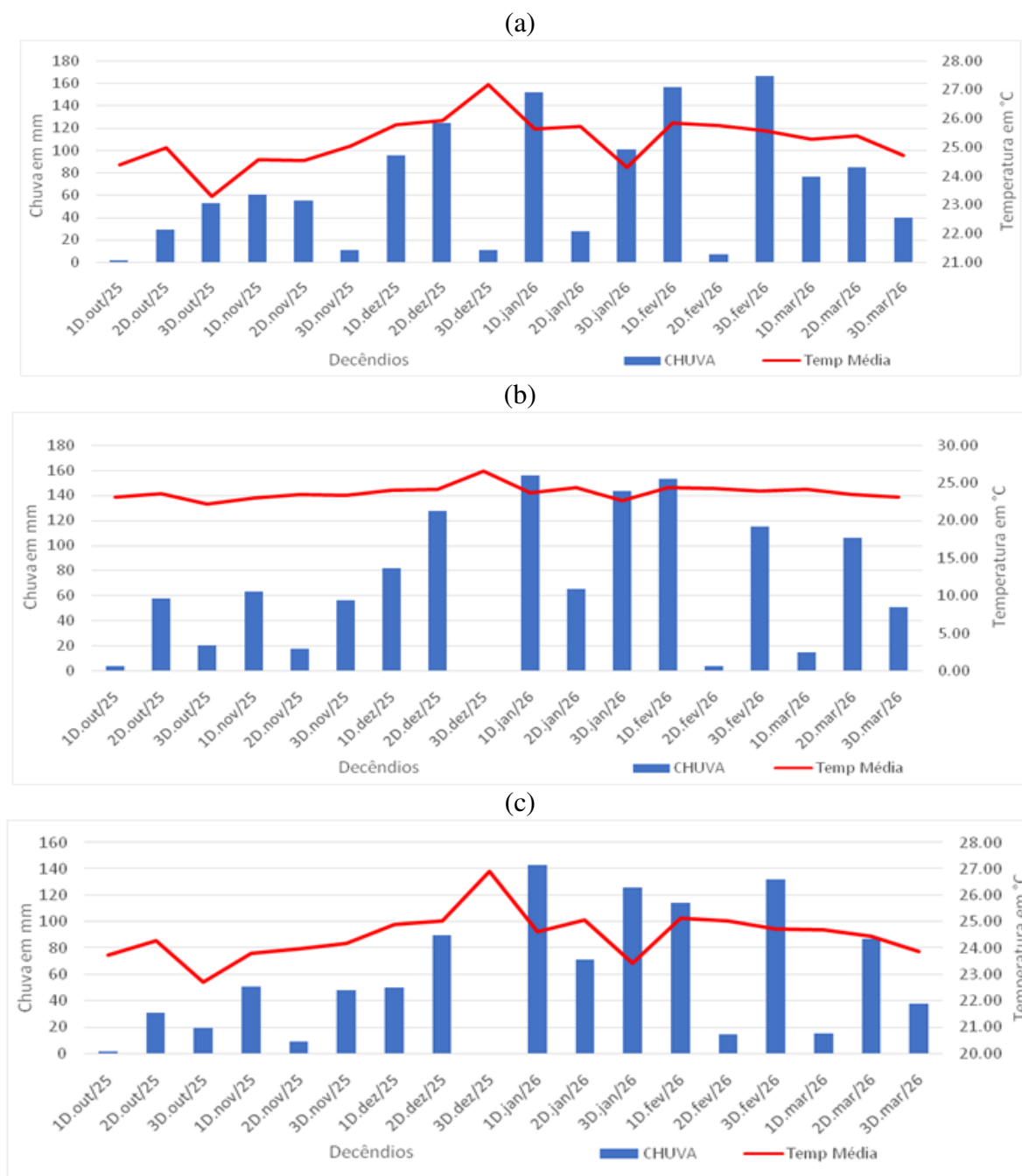
Figura 3: Histograma de Chuva e Temperatura: Caratinga (a); Timóteo (b) e PERD (c) – (outubro de 2025 a março de 2026).
