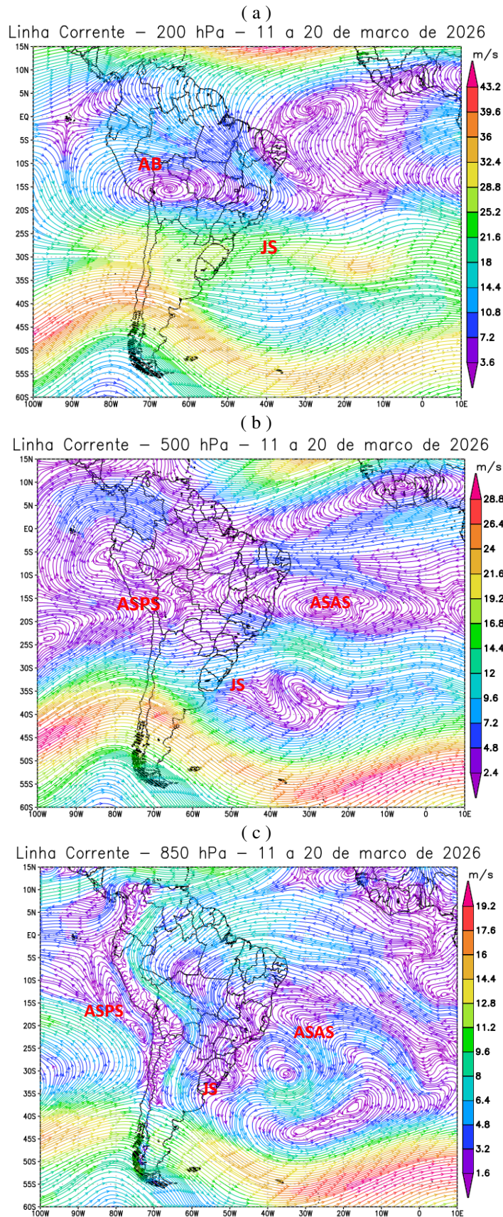
Figura 7 - Campos de Linha de Corrente 200 hPa (a), 500 hPa (b) e 850 hPa (c), do 2º Decêndio de março de 2026; demonstrando interação entre os sistemas atmosféricos: Jato Subtropical (JS), Alta da Bolívia (AB), Anticiclone Subtropical do Atlântico Sul (ASAS) e o Anticiclone Subtropical do Pacífico Sul (ASPS). FONTE - Dados: ECMWF 2026.
