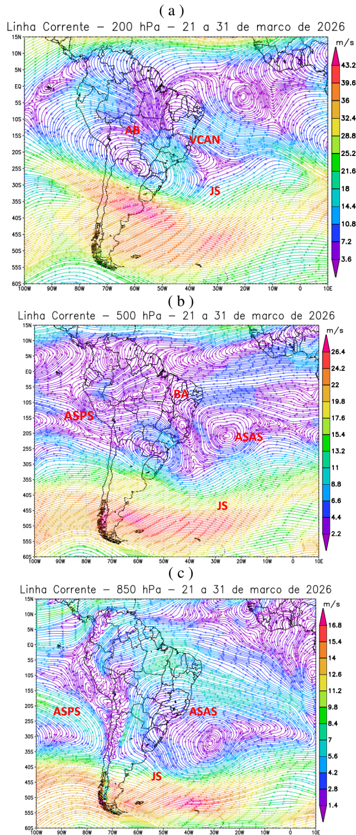
Figura 8 - Campos de Linha de Corrente 200 hPa (a), 500 hPa (b) e 850 hPa (c), do 3º Decêndio de março de 2026; demonstrando interação entre os sistemas atmosféricos: Jato Subtropical (JS), Alta da Bolívia, Vórtice Ciclônico de Altos Níveis (VCAN), Bloqueio Atmosférico (BA), Anticiclone Subtropical do Atlântico Sul (ASAS) e Anticiclone Subtropical do Pacífico Sul (ASPS).
