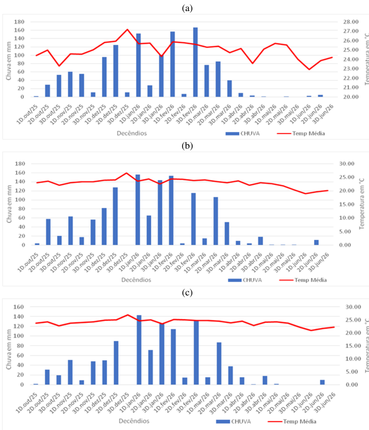
Figura 3: Histograma de Chuva e Temperatura: Caratinga (a); Timóteo (b) e PERD (c) – (outubro de 2025 a junho de 2026).
