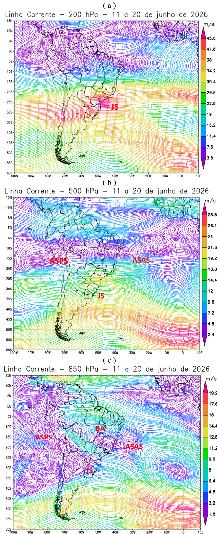
Figura 7 - Campos de Linha de Corrente 200 hPa (a), 500 hPa (b) e 850 hPa (c), do 2º Decêndio de junho de 2026; demonstrando interação entre os sistemas atmosféricos: Jato Subtropical (JS), Bloqueio Atmosférico (BA), Anticiclone Subtropical do Atlântico Sul (ASAS) e o Anticiclone Subtropical do Pacífico Sul (ASPS).
