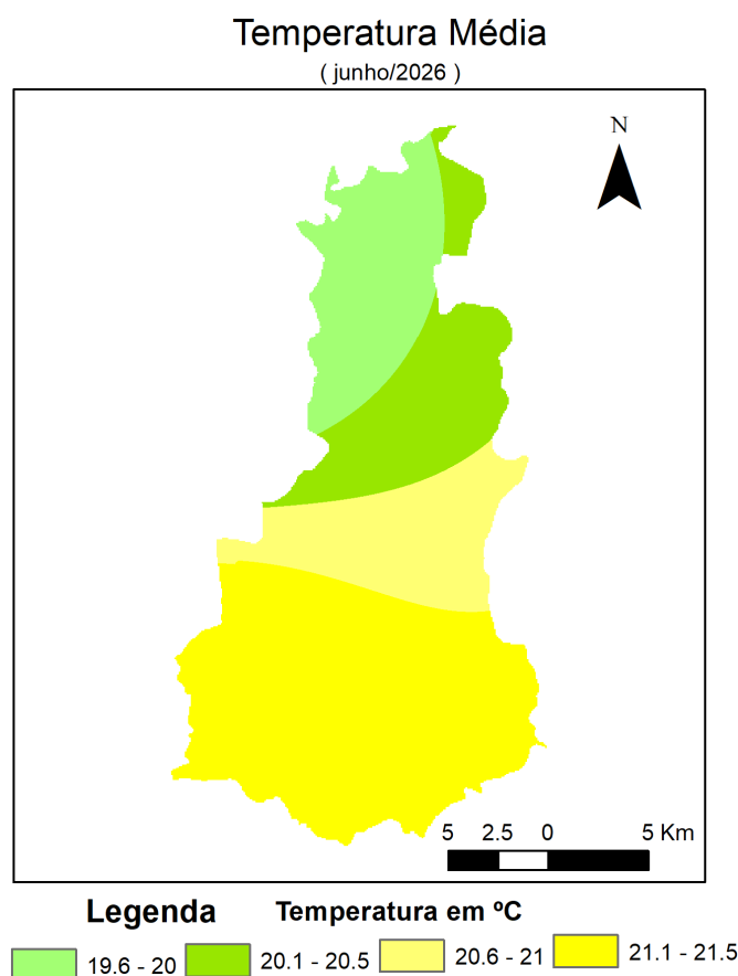
Figura 4 - Espacialização da Temperatura Média em junho de 2026. FONTE dos Dados: INMET e CEMADEN
