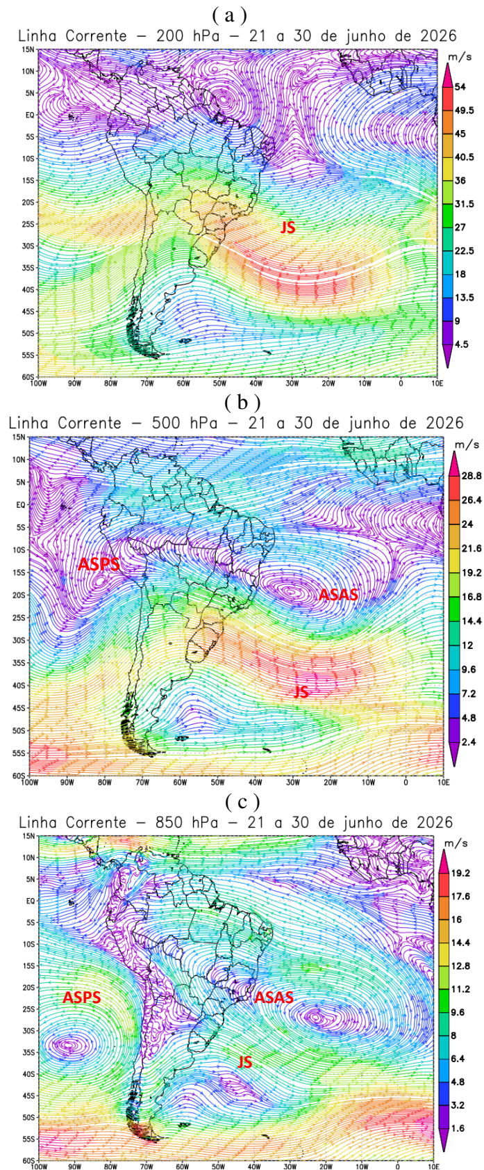
Figura 8 - Campos de Linha de Corrente 200 hPa (a), 500 hPa (b) e 850 hPa (c), do 3º Decêndio de junho de 2026; demonstrando interação entre os sistemas atmosféricos: Jato Subtropical (JS), Anticiclone Subtropical do Atlântico Sul (ASAS) e Anticiclone Subtropical do Pacífico Sul (ASPS).
