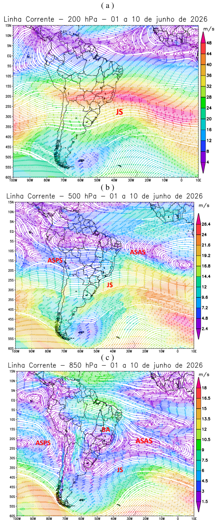
Figura 6 - Campos de Linha de Corrente 200 hPa (a), 500 hPa (b) e 850 hPa (c), do 1º Decêndio de junho de 2026; demonstrando interação entre os sistemas atmosféricos: Jato Subtropical (JS), Bloqueio Atmosférico (BA), Anticiclone Subtropical do Atlântico Sul (ASAS) e o Anticiclone Subtropical do Pacífico Sul (ASPS). FONTE - Dados: ECMWF 2026.
