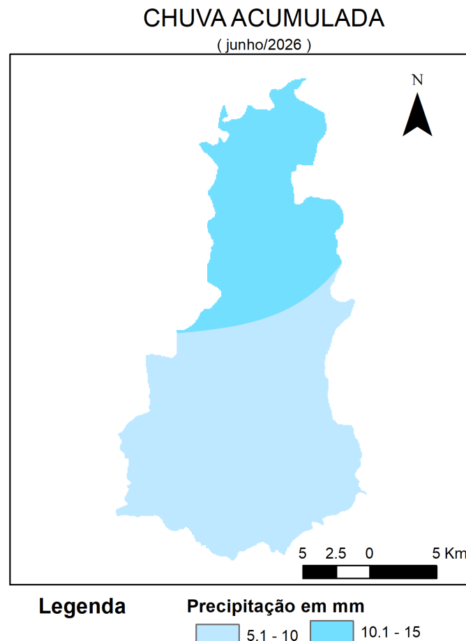
Figura 5 - Espacialização da Chuva da Acumulada em junho de 2026. FONTE dos Dados: INMET e CEMADEN
