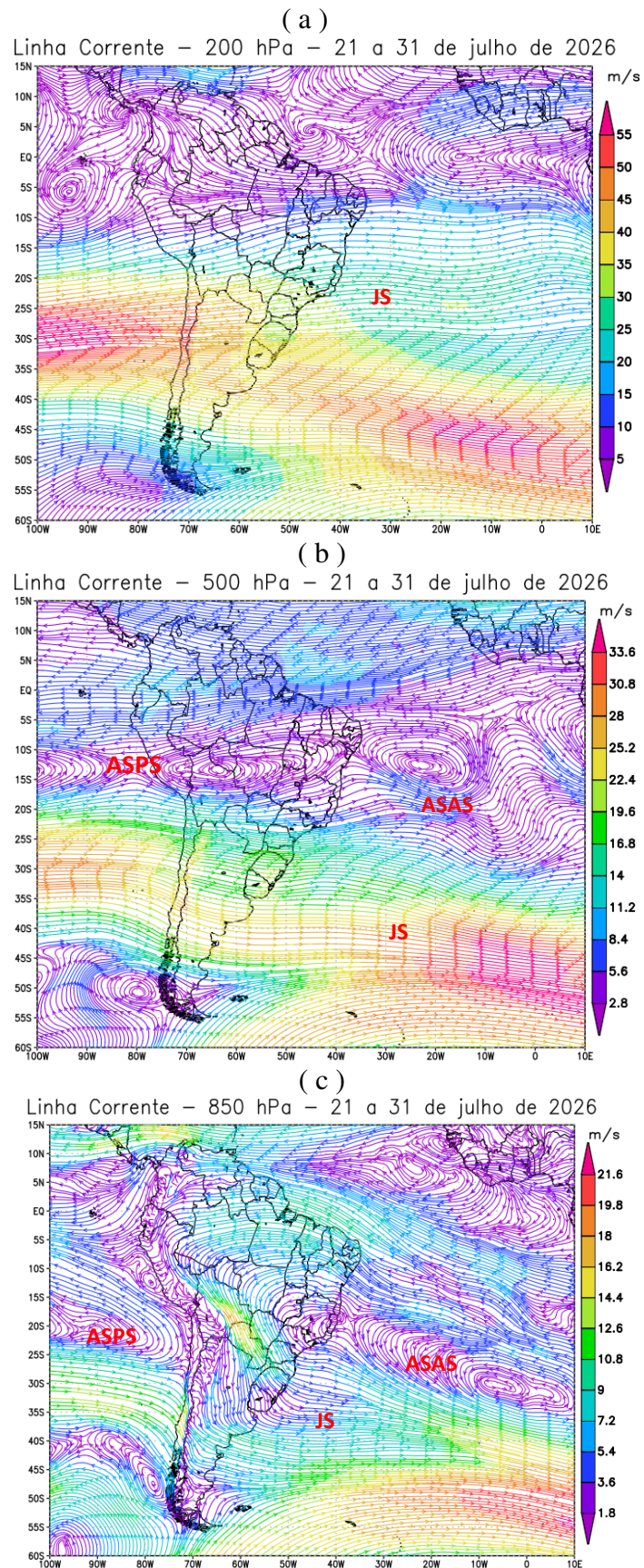
Figura 8 - Campos de Linha de Corrente 200 hPa (a), 500 hPa (b) e 850 hPa (c), do 3º Decêndio de julho de 2026; demonstrando interação entre os sistemas atmosféricos: Jato Subtropical (JS), Anticiclone Subtropical do Atlântico Sul (ASAS) e Anticiclone Subtropical do Pacífico Sul (ASPS).
