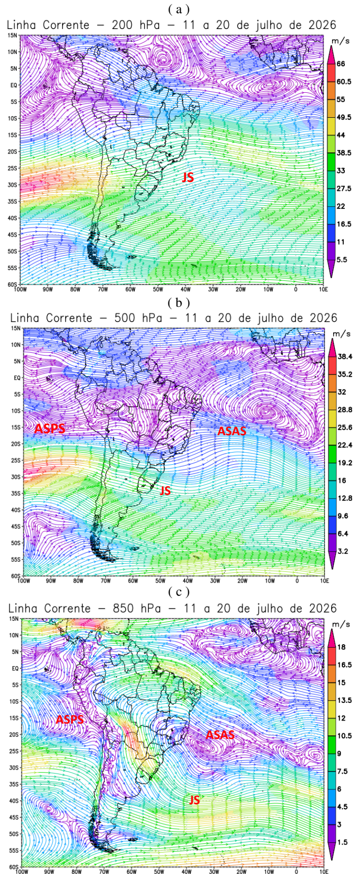
Figura 7 - Campos de Linha de Corrente 200 hPa (a), 500 hPa (b) e 850 hPa (c), do 2º Decêndio de julho de 2026; demonstrando interação entre os sistemas atmosféricos: Jato Subtropical (JS), Anticiclone Subtropical do Atlântico Sul (ASAS) e o Anticiclone Subtropical do Pacífico Sul (ASPS).
