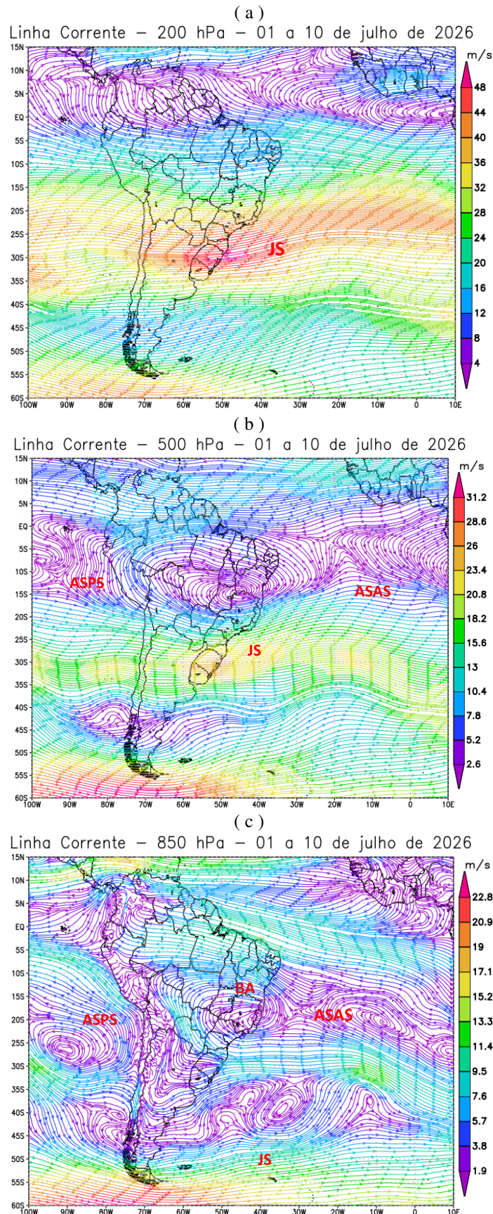
Figura 6 - Campos de Linha de Corrente 200 hPa (a), 500 hPa (b) e 850 hPa (c), do 1º Decêndio de julho de 2026; demonstrando interação entre os sistemas atmosféricos: Jato Subtropical (JS), Bloqueio Atmosférico (BA), Anticiclone Subtropical do Atlântico Sul (ASAS) e o Anticiclone Subtropical do Pacífico Sul (ASPS).
