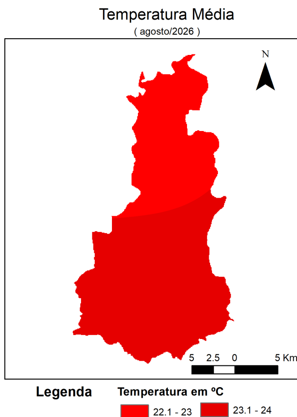
Figura 4 - Espacialização da Temperatura Média em agosto de 2026. FONTE dos Dados: INMET e CEMADEN
