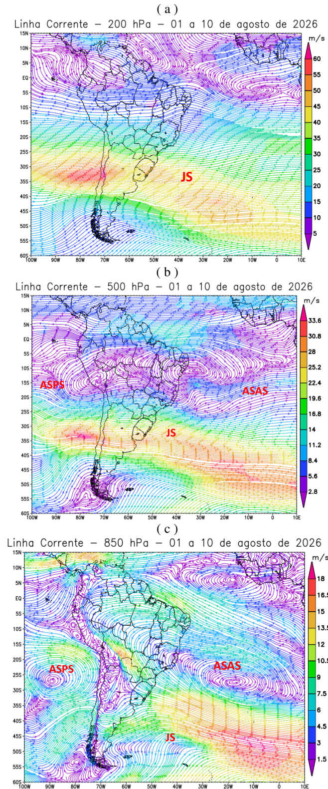
Figura 6 - Campos de Linha de Corrente 200 hPa (a), 500 hPa (b) e 850 hPa (c), do 1º Decêndio de agosto de 2026; demonstrando interação entre os sistemas atmosféricos: Jato Subtropical (JS), Anticiclone Subtropical do Atlântico Sul (ASAS) e o Anticiclone Subtropical do Pacífico Sul (ASPS).
