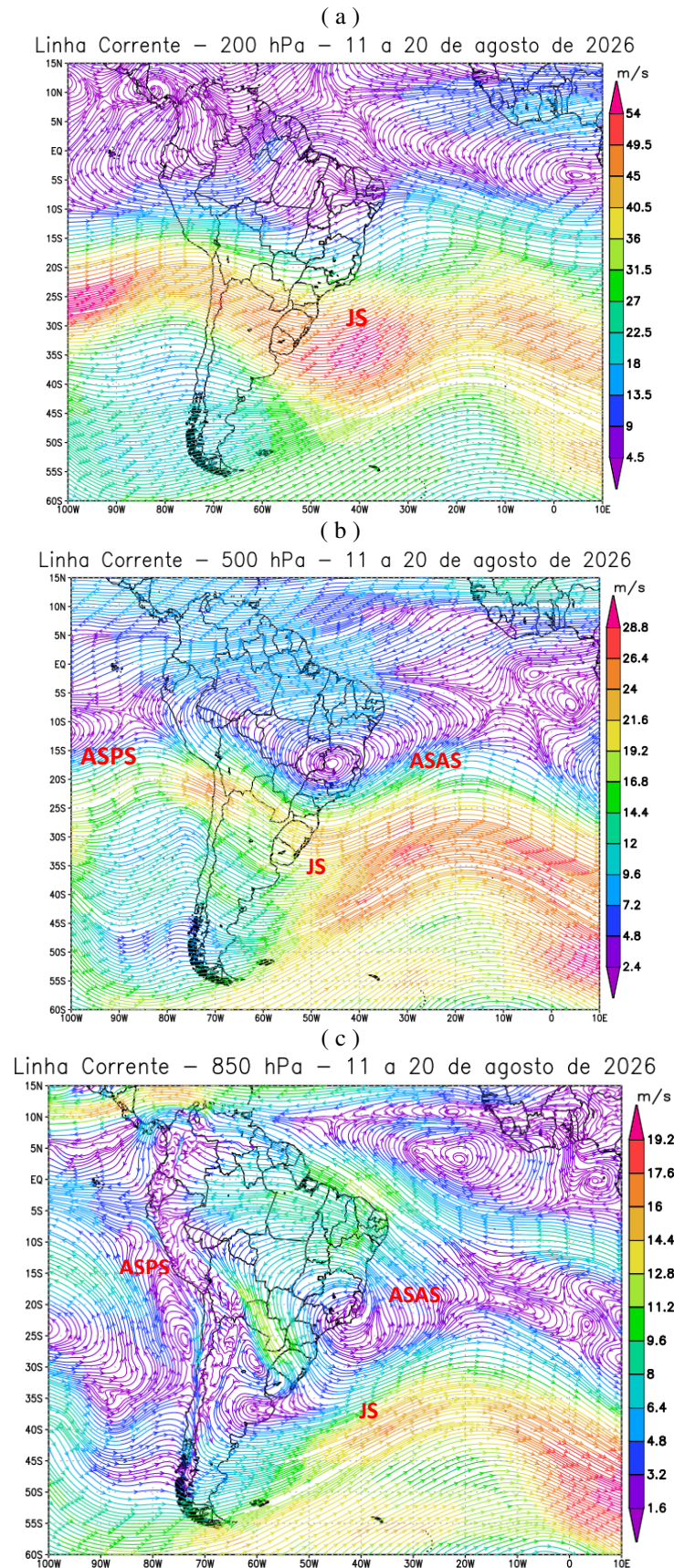
Figura 7 - Campos de Linha de Corrente 200 hPa (a), 500 hPa (b) e 850 hPa (c), do 2º Decêndio de agosto de 2026; demonstrando interação entre os sistemas atmosféricos: Jato Subtropical (JS), Anticiclone Subtropical do Atlântico Sul (ASAS) e o Anticiclone Subtropical do Pacífico Sul (ASPS).
