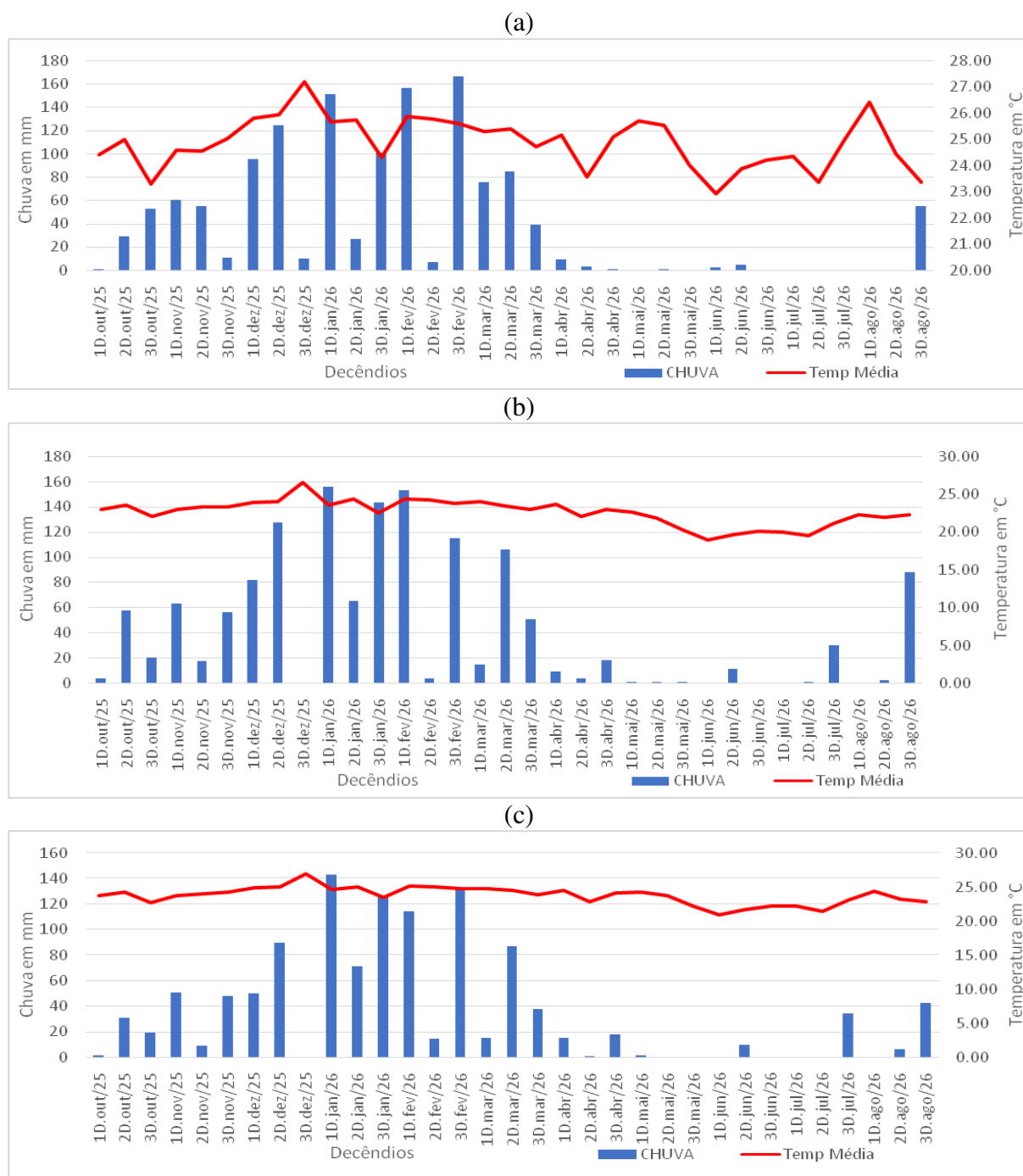
Figura 3: Histograma de Chuva e Temperatura: Caratinga (a); Timóteo (b) e PERD (c) – (outubro de 2025 a agosto de 2026).
