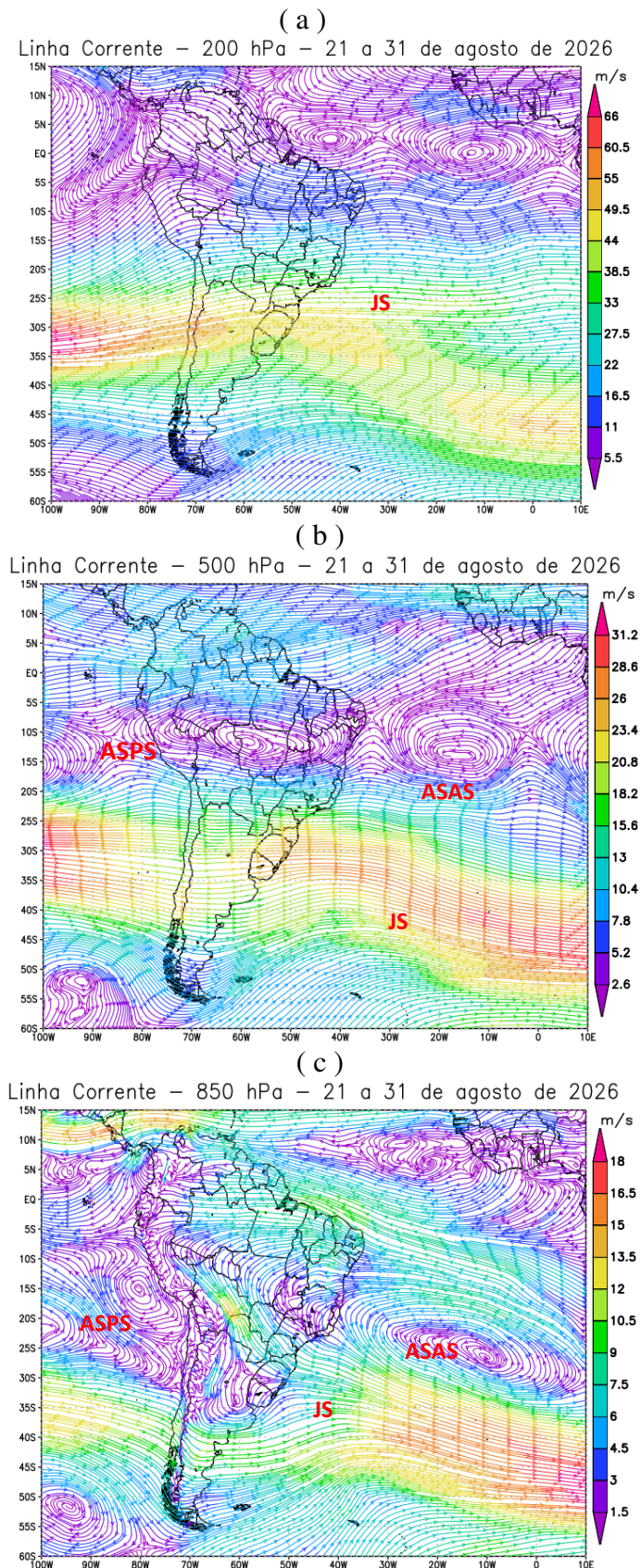
Figura 8 - Campos de Linha de Corrente 200 hPa (a), 500 hPa (b) e 850 hPa (c), do 3º Decêndio de agosto de 2026; demonstrando interação entre os sistemas atmosféricos: Jato Subtropical (JS), Anticiclone Subtropical do Atlântico Sul (ASAS) e Anticiclone Subtropical do Pacífico Sul (ASPS).
