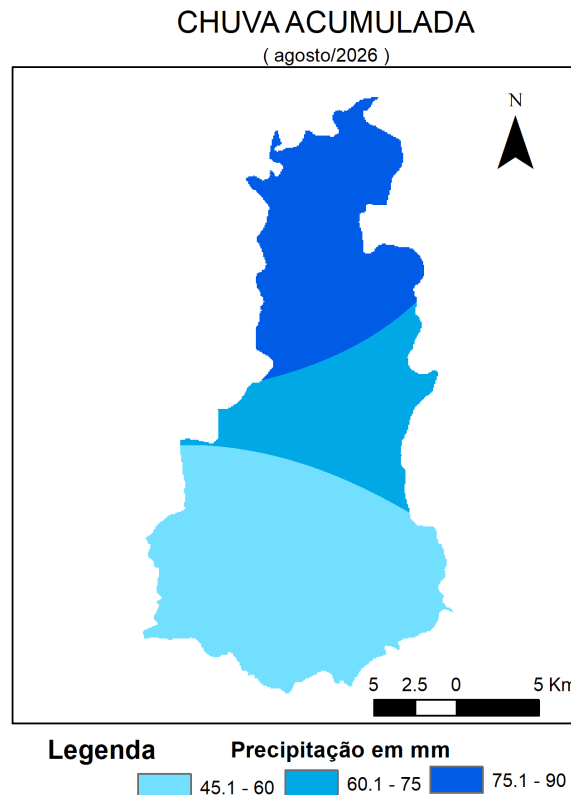
Figura 5 - Espacialização da Chuva da Acumulada em agosto de 2026. FONTE dos Dados: INMET e CEMADEN
