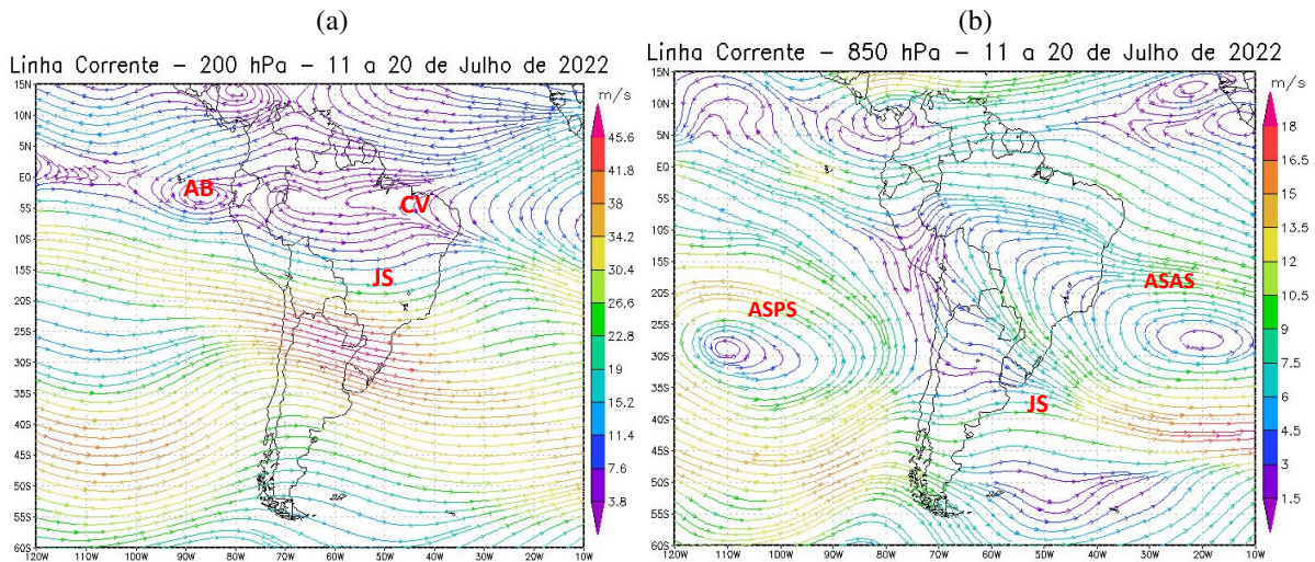
Figura 7 - Campos de Linha de Corrente 200 hPa. - (a) e 850 hPa. - (b), do 2º Decêndio de julho de 2022; demonstrando interação entre os sistemas atmosféricos: Jato Subtropical (JS), Alta da Bolívia (AB), Anticiclone Subtropical do Atlântico Sul (ASAS) e o Anticiclone Subtropical do Pacífico Sul (ASPS) e Cavado (CV).
