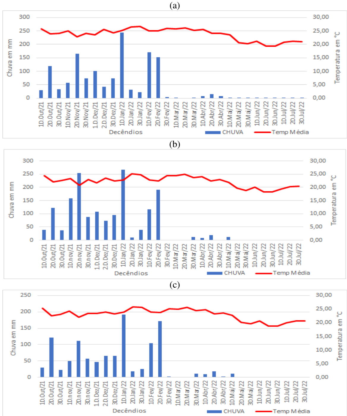
Figura 3: Histograma de Chuva e Temperatura: Caratinga (a); Timóteo (b) e PERD (c) – (outubro de 2021 a julho de 2022).
