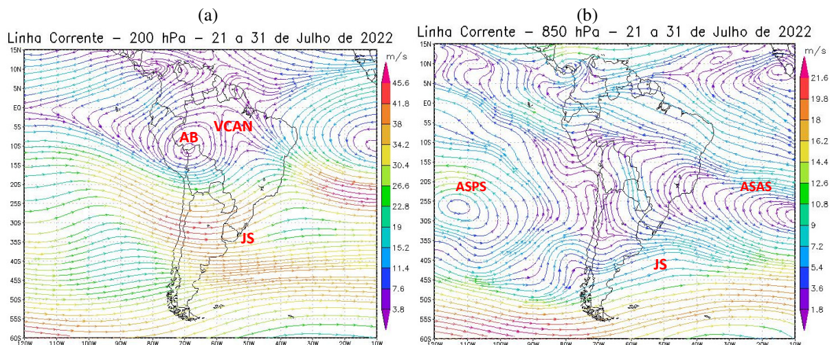
Figura 8 - Campos de Linha de Corrente 200 hPa. - (a) e 850 hPa. - (b), do 3º Decêndio de julho de 2022; demonstrando interação entre os sistemas atmosféricos: Jato Subtropical (JS), Alta da Bolívia (AB), Anticiclone Subtropical do Atlântico Sul (ASAS) e o Anticiclone Subtropical do Pacífico Sul (ASPS) e Vórtice Ciclônico de Altos Níveis (VCAN).
