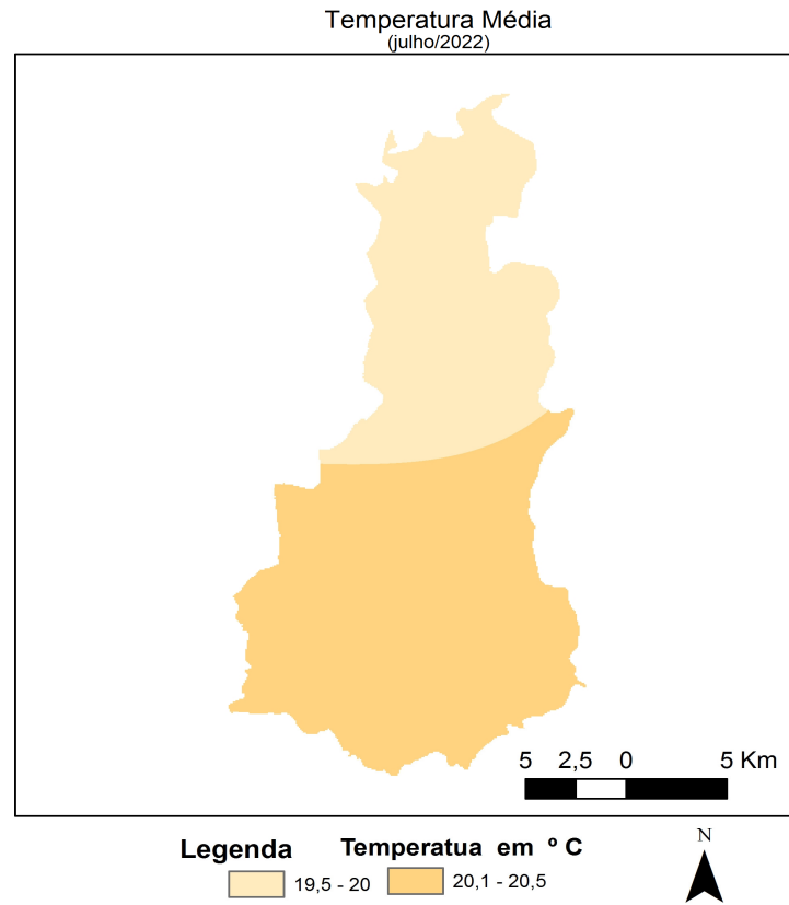
Figura 4 - Espacialização da Temperatura Média em julho de 2022. FONTE dos Dados: INMET e INPE
