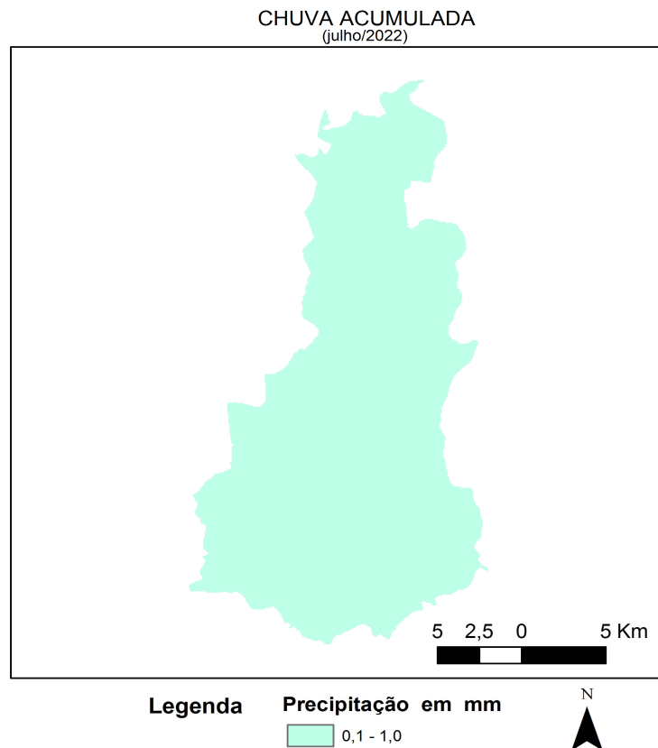
Figura 5 - Espacialização da Chuva da Acumulada em julho de 2022. FONTE dos Dados: INMET e INPE
