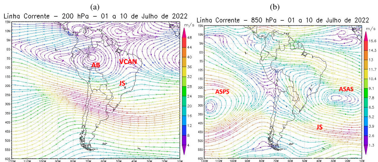
Figura 6 - Campos de Linha de Corrente 200 hPa. - (a) e 850 hPa. - (b), do 1º Decêndio de julho de 2022; demonstrando interação entre os sistemas atmosféricos: Jato Subtropical (JS), Alta da Bolívia (AB), Anticiclone Subtropical do Atlântico Sul (ASAS) e o Anticiclone Subtropical do Pacífico Sul (ASPS) e Vórtice Ciclônico de Altos Níveis (VCAN). FONTE - Dados: NOAA 2022.
