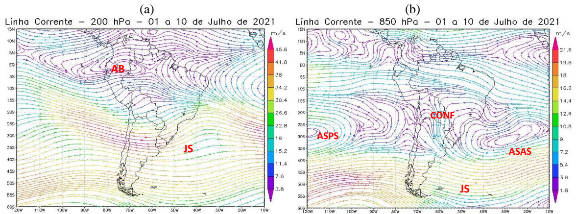
Figura 6 - Campos de Linha de Corrente 200 hPa. - (a) e 850 hPa. - (b), do 1º Decêndio de julho de 2021; demonstrando interação entre os sistemas atmosféricos: Confluência (CONF), Alta da Bolívia (AB), Jato Subtropical (JS), Anticiclone Subtropical do Atlântico Sul (ASAS) e o Anticiclone Subtropical do Pacífico Sul (ASPS).
