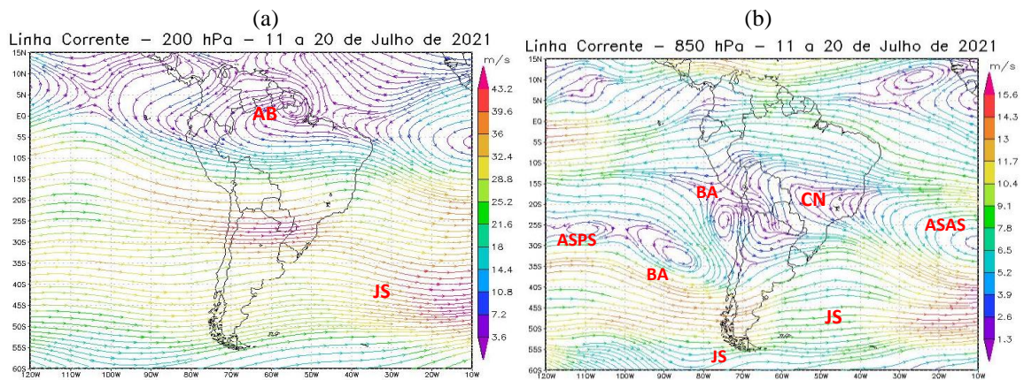
Figura 7 - Campos de Linha de Corrente 200 hPa. - (a) e 850 hPa. - (b), do 2º Decêndio de julho de 2021; demonstrando interação entre os sistemas atmosféricos: Alta da Bolívia (AB), Jato Subtropical (JS), Bloqueio Atmosférico (BA), Cavado do Nordeste (CN), Anticiclone Subtropical do Atlântico Sul (ASAS) e o Anticiclone Subtropical do Pacífico Sul (ASPS).
