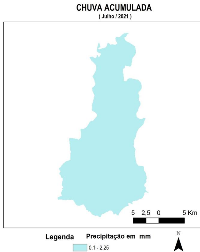
Figura 5 - Espacialização da Chuva da Acumulada em julho de 2021. FONTE dos Dados: INMET e INPE
