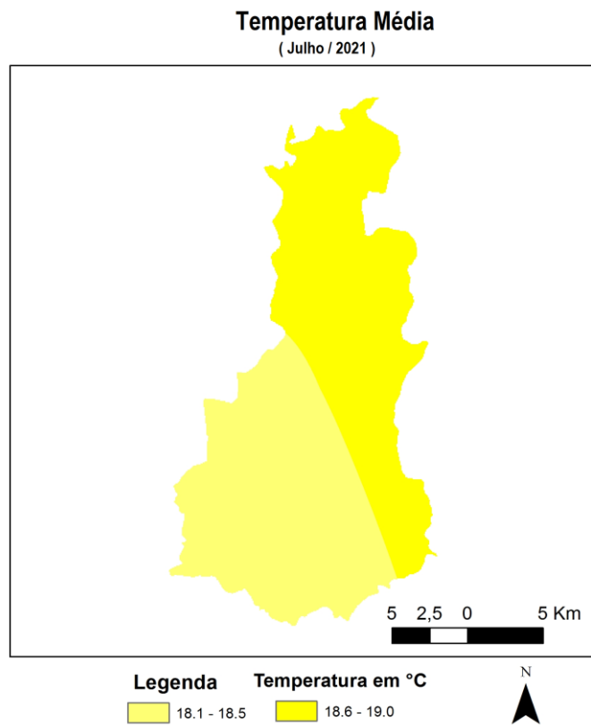
Figura 4 - Espacialização da Temperatura Média em julho de 2021. FONTE dos Dados: INMET e INPE
