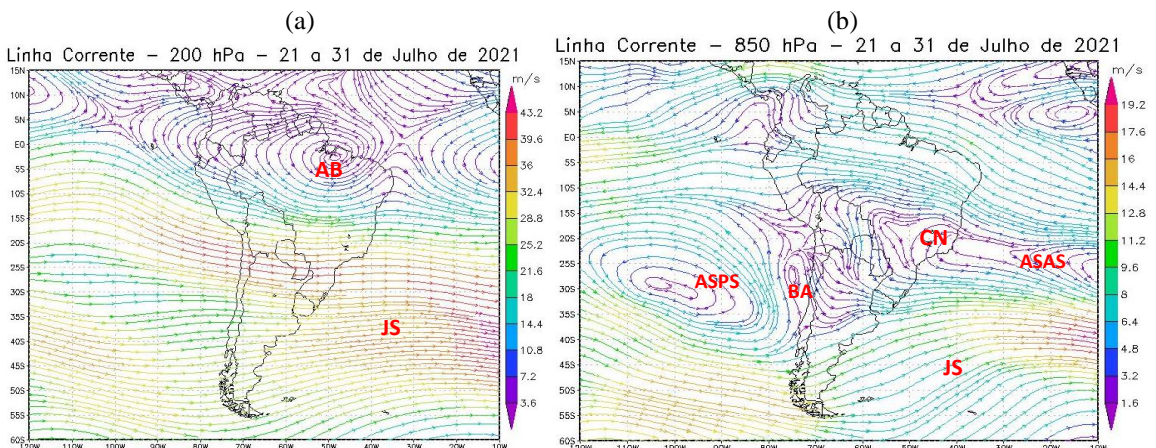
Figura 8 - Campos de Linha de Corrente 200 hPa. - (a) e 850 hPa. - (b), do 3º Decêndio de julho de 2021; demonstrando interação entre os sistemas atmosféricos: Alta da Bolívia (AB), Jato Subtropical (JS), Bloqueio Atmosférico (BA), Cavado do Nordeste (CN), Anticiclone Subtropical do Atlântico Sul (ASAS) e o Anticiclone Subtropical do Pacífico Sul (ASPS).
