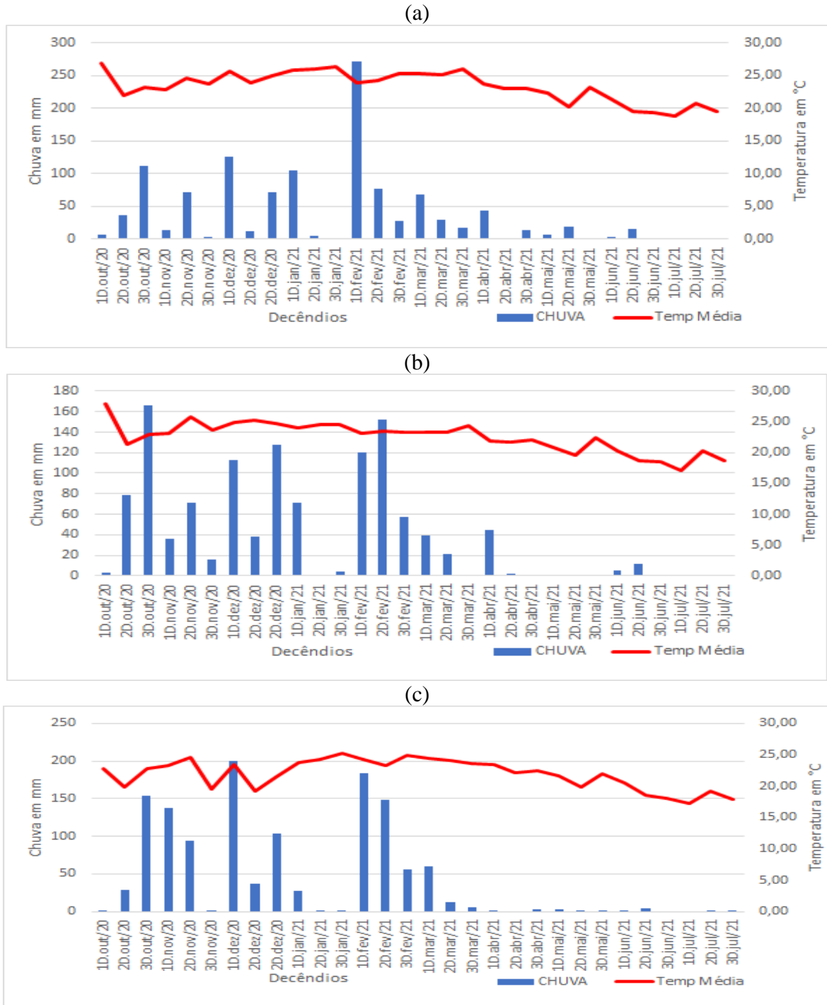
Figura 3: Histograma de Chuva e Temperatura: Caratinga (a); Timóteo (b) e PERD (c) – (outubro/2020 a julho/2021).
