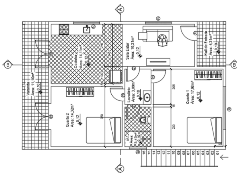
Figura 1 – Planta Baixa Projeto Original, 2023
