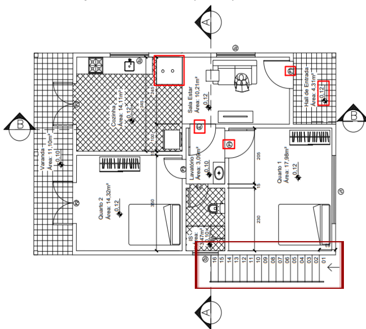
Figura 2 – Planta Baixa Projeto Modificado, 2023
